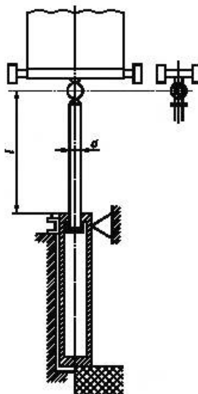
Рисунок 11— Гидроцилиндры одиночного действия
