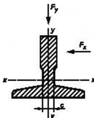
Рисунок 1 — Профиль направляющей
