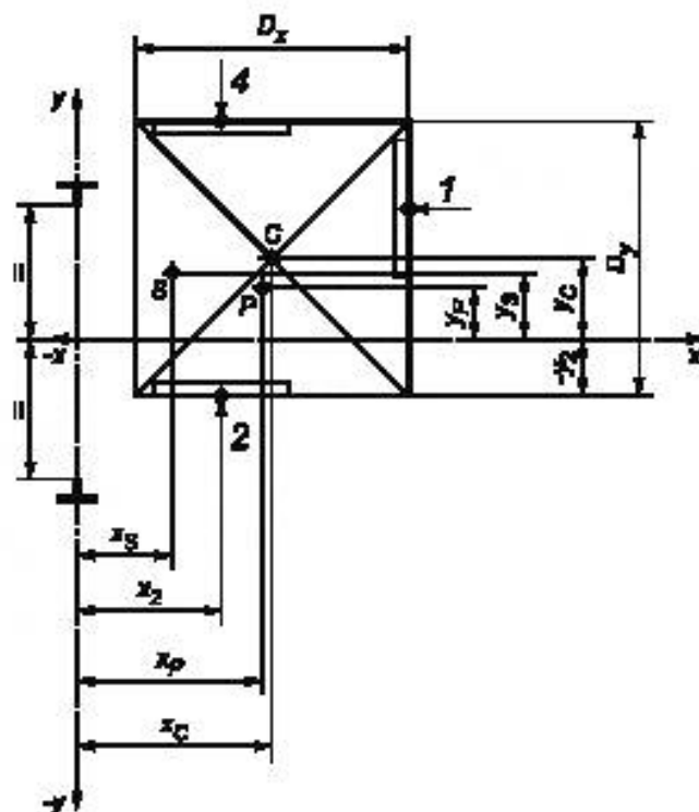
Рисунок А.4 — Режим нормальной работы. Загрузка
