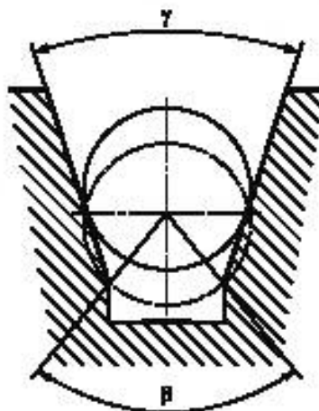
Рисунок 4 — Клиновая канавка с подрезом
