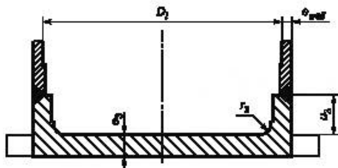
Рисунок 10 — Плоское основание со сварным фланцем
