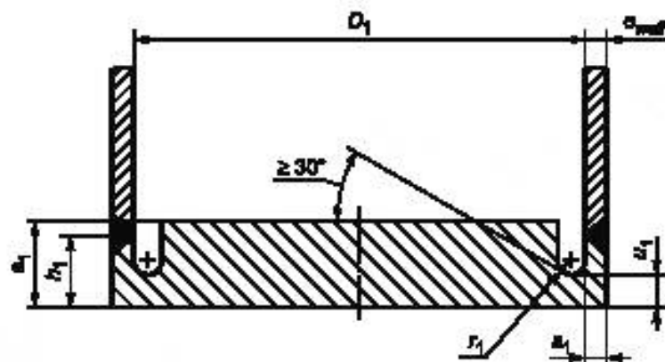
Рисунок 8 — Плоские основания с разгрузочной канавкой
