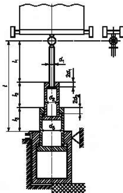
Рисунок 12 — Телескопические гидроцилиндры без внешней направляющей
