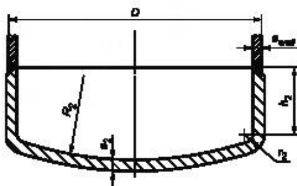
Рисунок 9 — Выгнутое основание
