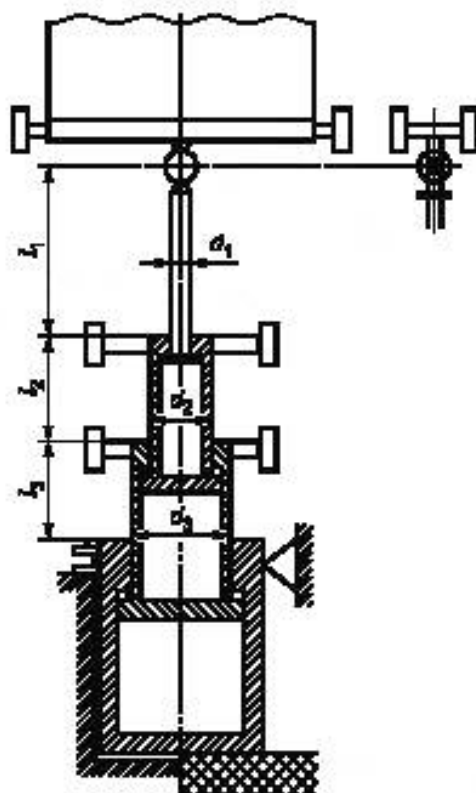
Рисунок 13 — Телескопические гидроцилиндры с внешней направляющей
