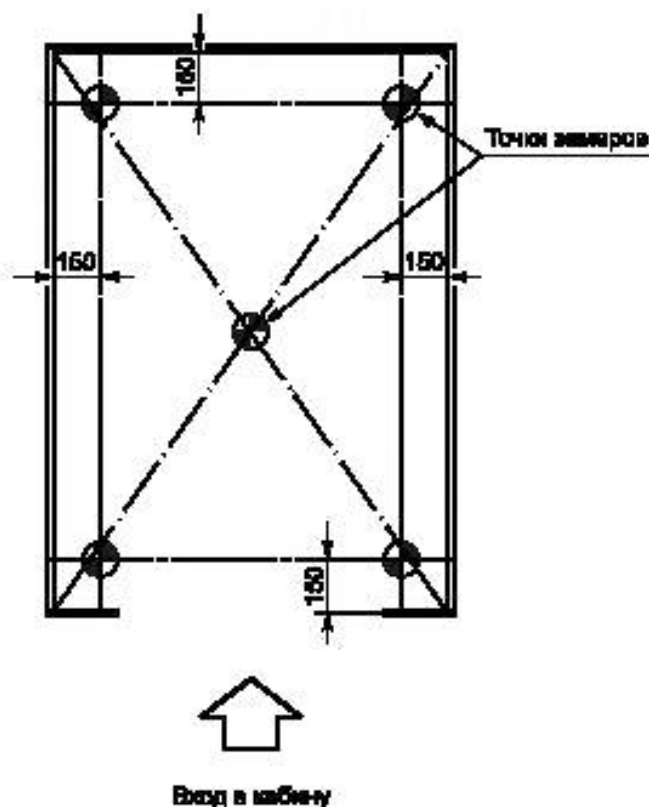
Рисунок ДБ.1 — Схема расположения контрольных точек
