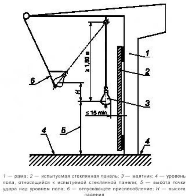
Рисунок ДД.3 — Высота падения
