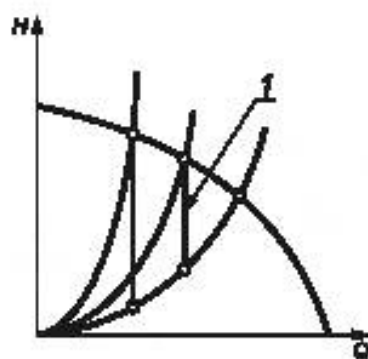
Рисунок F.2 — Примеры уровня расхода при дросселировании задвижки
