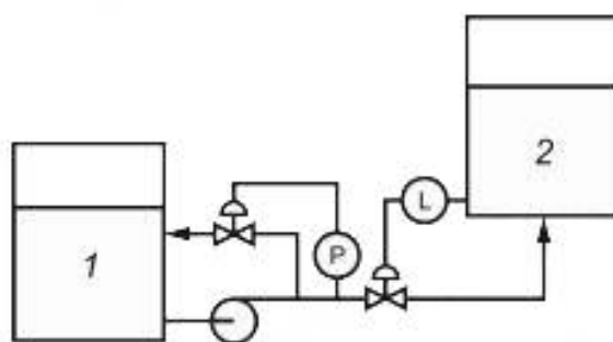
Рисунок В.3 — Пример упрощенной технологической схемы
