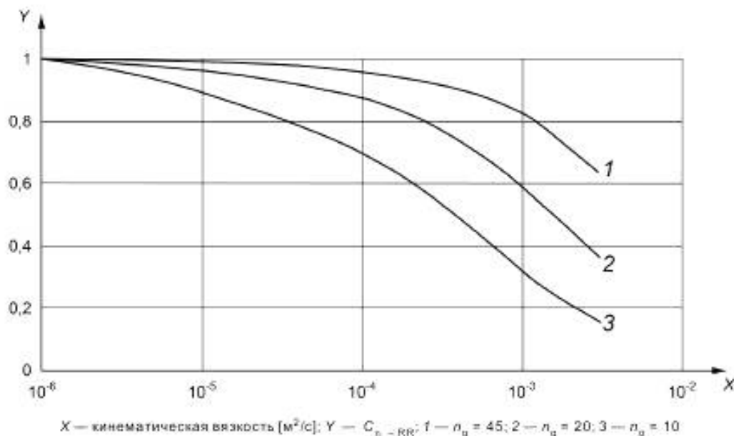
Рисунок Б.2 — Влияние дисковых потерь на КПД
