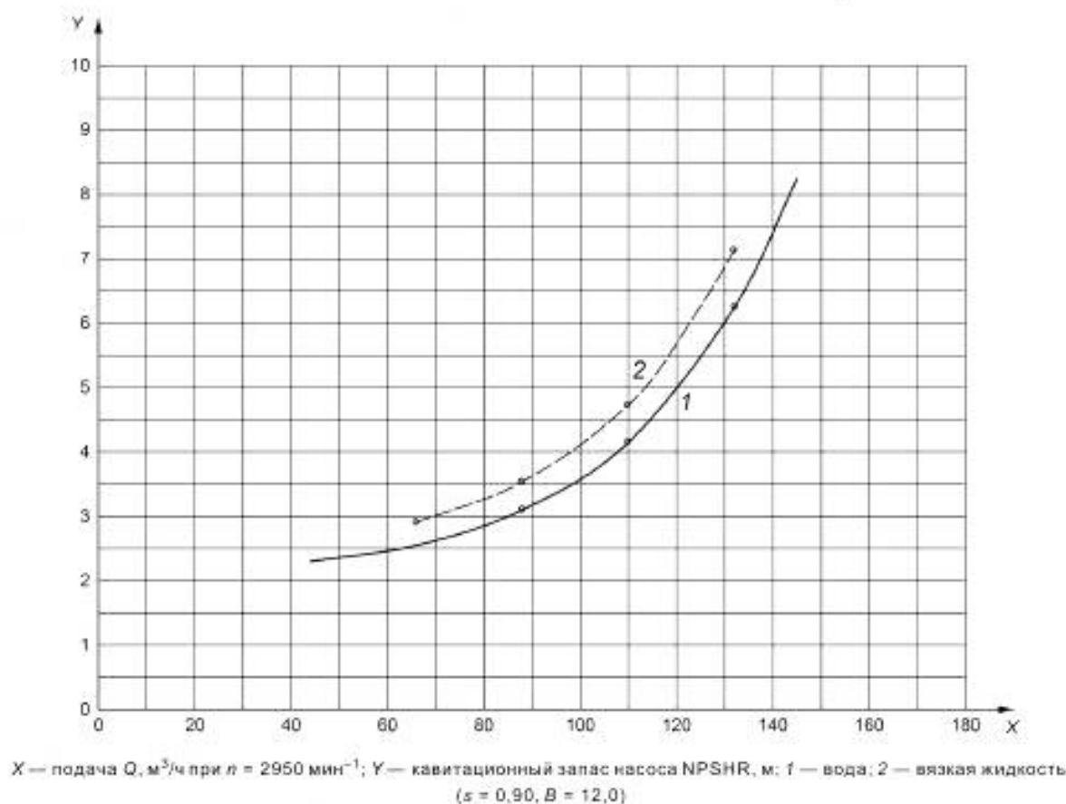
Рисунок Б.3 — Результат пересчета NPSHR
