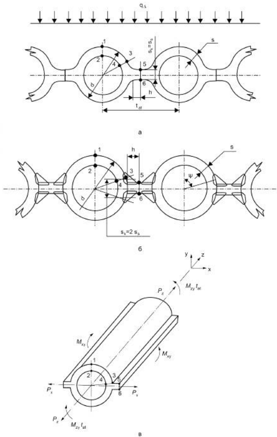
а — мембранный экран из плавниковых труб; б — мембранный экран из гладких труб; в — схема приложения усилий и моментов к ребренной трубе
