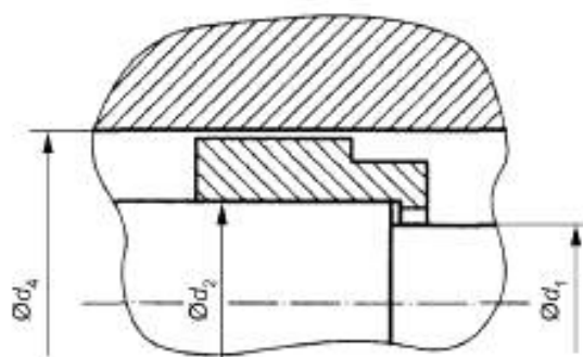
Рисунок 2 — Разгруженное торцовое уплотнение с короткой втулкой
