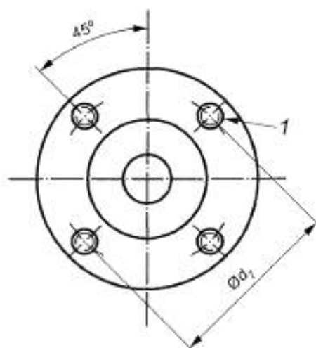
Рисунок 5 — Крышка корпуса уплотнения (отверстия под крепеж)
