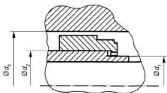
Рисунок 3 — Разгруженное торцовое уплотнение с длинной втулкой
