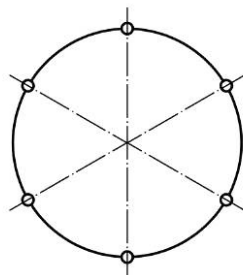
Рисунок 4 — Пример установки тензодатчика в шести точках (три комплекта) с шагом 60°
