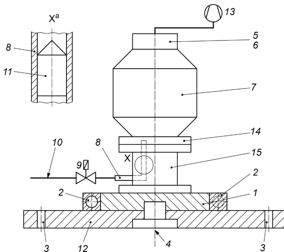
Рисунок 8 — Схема оборудования для проведения разрушающего контроля методом С «столкновение с препятствием»
