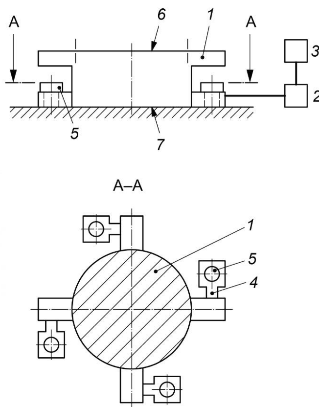
1 — стенд; 2 — усилитель тензодатчиков или датчиков силы; 3 — регистрирующее устройство; 4 — стержни, работающие на сжатие, с тензодатчиками или с датчиками силы; 5 — анкерные болты; 6 — поверхность насоса; 7 — сторона крепления
