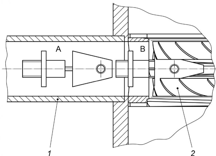
A — снаряд в положении покоя; B — снаряд в заданной точке 1 — пусковое устройство; 2 — турбомолекулярный насос (лопатки ротора)
