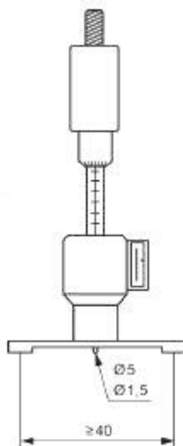
Рисунок 7 — Микрометр с добавочным приспособлением для измерения глубины вмятины, вызванной индентором при ударе
