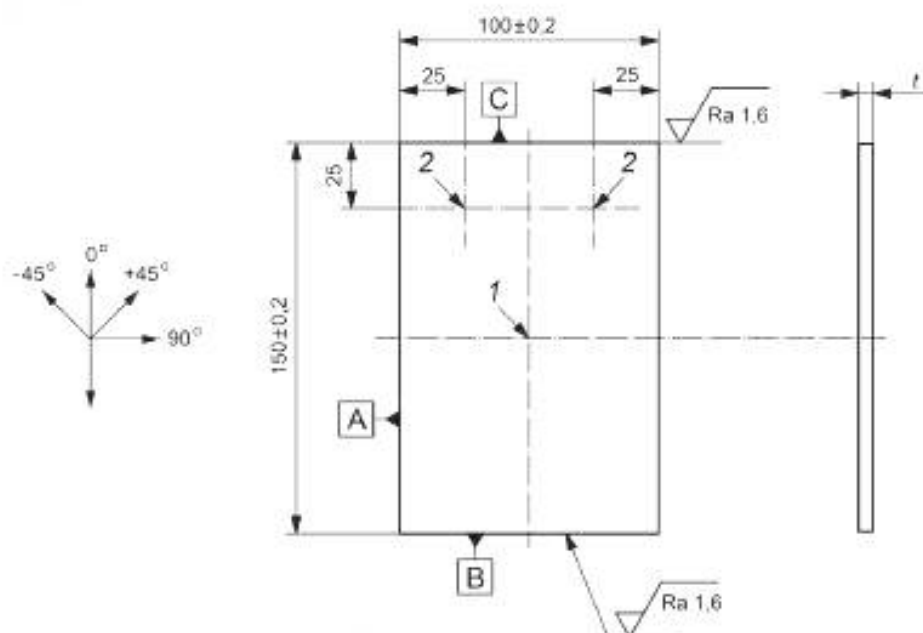
Рисунок 8 — Форма и размеры образца для испытаний и расположение тензометров
