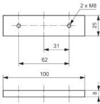
Рисунок А.6 — Основные размеры верхней зажимной плиты
