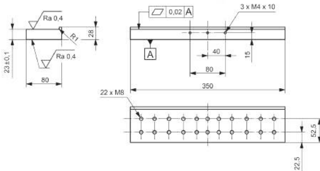
Рисунок А.1 — Конфигурация и размеры опоры
