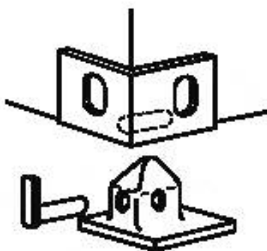
Рисунок 8 – Штыковой упор с закладным пальцем
