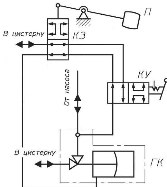
Рисунок А.1 — Гидравлическая принципиальная схема ограничителя наполнения
