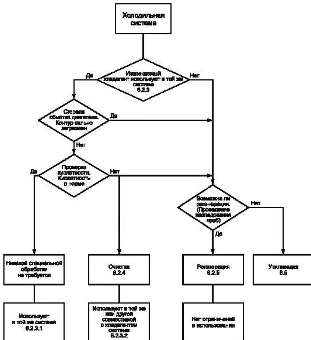
Рисунок 2 — Блок-схема операций, выполняемых при извлечении хладагента
