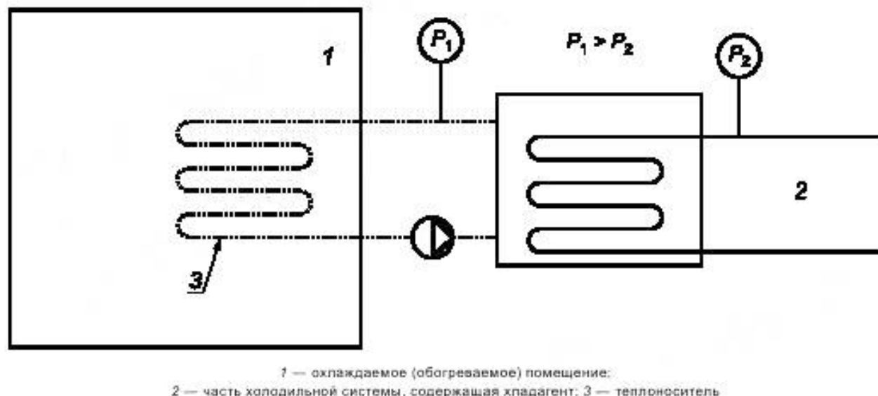
Рисунок 9 — Промежуточная система высокого давления
