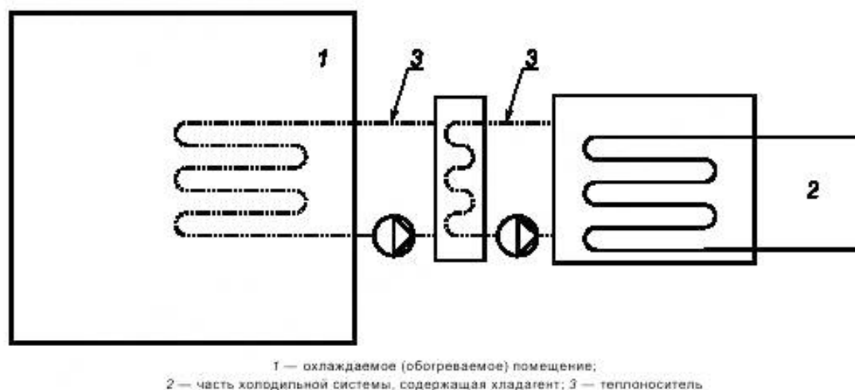
Рисунок 8 — Промежуточная сдвоенная система
