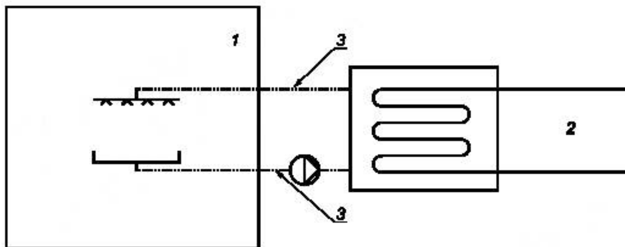
Рисунок 2 — Открытая оросительная система
