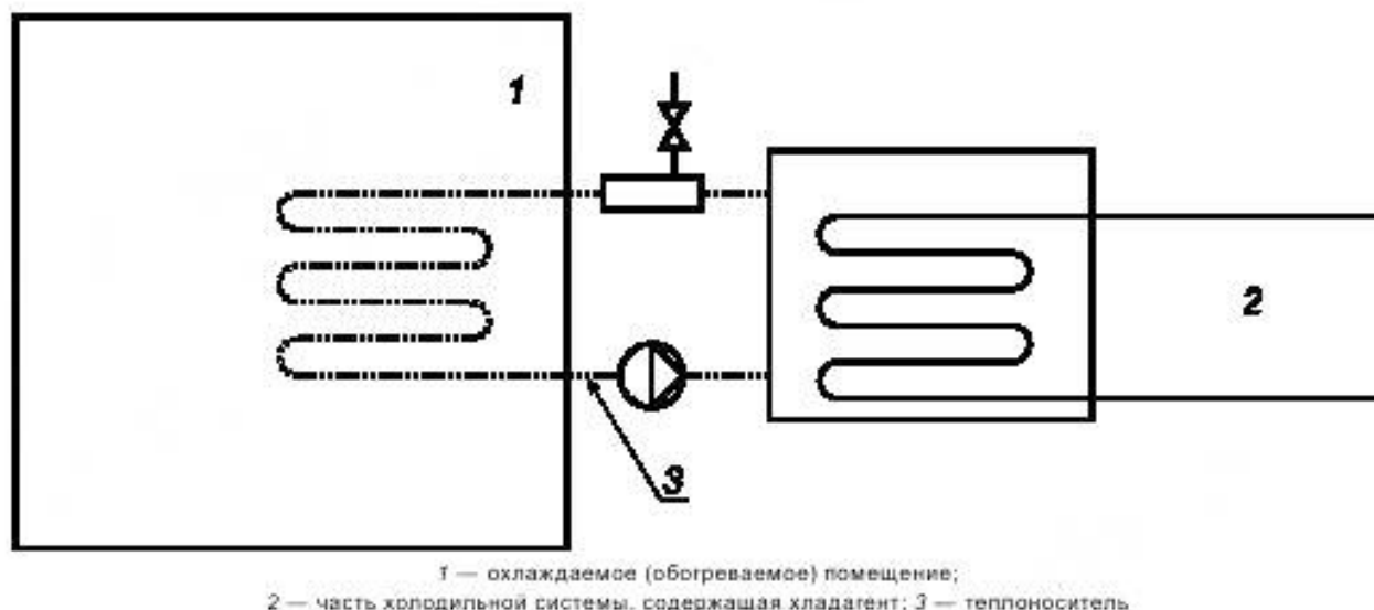
Рисунок 7 — Закрытая промежуточная система с вытяжкой
