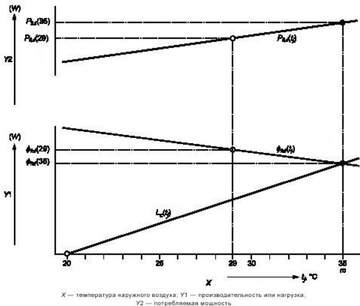
Рисунок А.1 — Холодопроизводительность, потребляемая мощность и нагрузка охлаждения для установок с нерегулируемой производительностью
