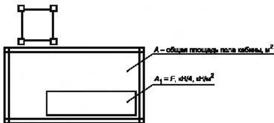
Рисунок 1 — Пример нагрузки в соответствии с 5.2.2.4 а)
