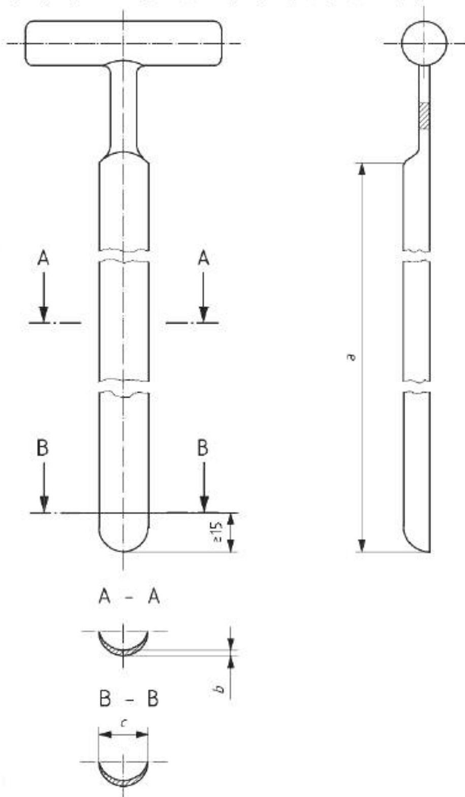
Рисунок А.1 – Щуп для сыра
