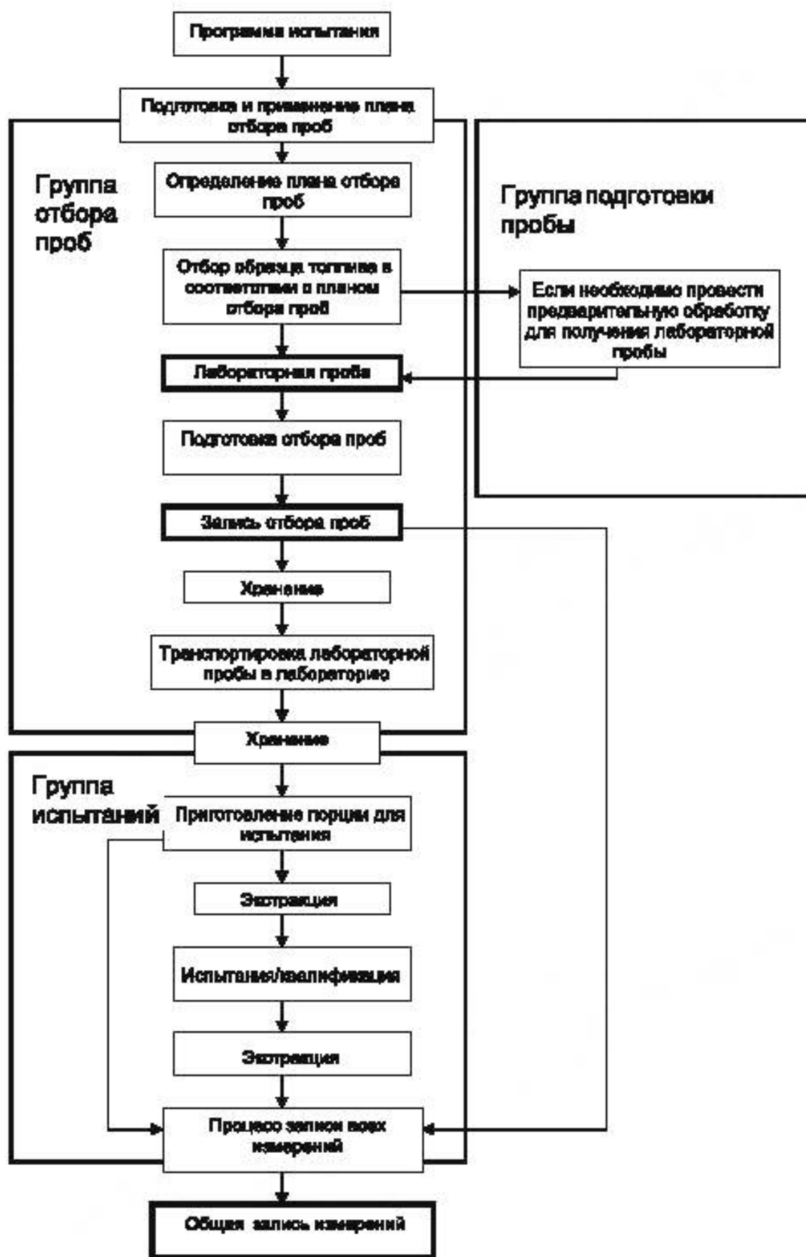
Рисунок 1 — Связи между существенными элементами программы испытаний
