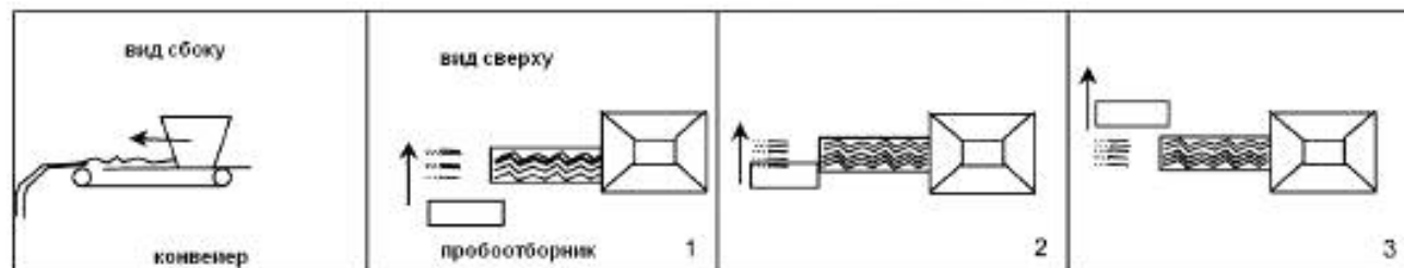
Рисунок Б.3 — Схематическое изображение отбора проб с конвейера
