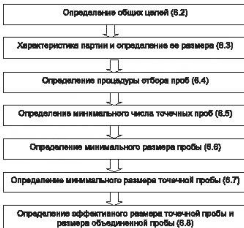
Рисунок 2 — Необходимые элементы для создания плана отбора проб
