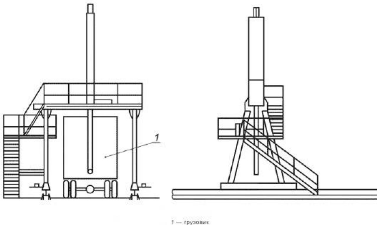
Рисунок Ж.9 — Пример механического пробоотборника
