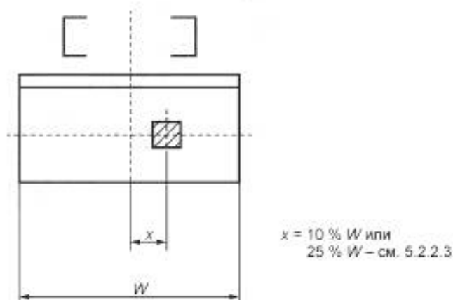
Рисунок 1 – Номинальная грузоподъемность при смещении от центра
