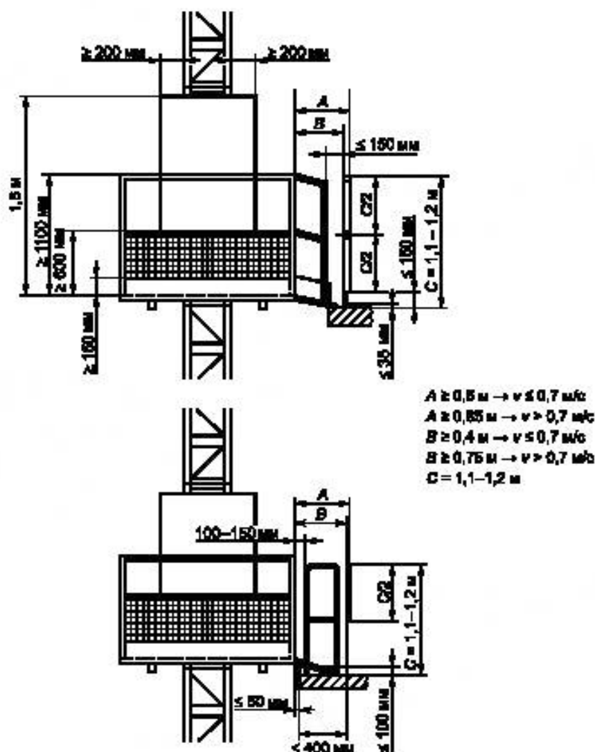
Рисунок 6 — Пример дверей погрузочной площадки уменьшенной высоты
