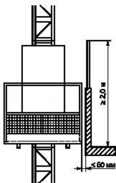
Рисунок 8 — Пример погрузочной площадки с неподвижным защитным устройством и дверью
