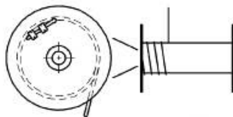
Рисунок 13 — Способы заделки концов проволочного каната
