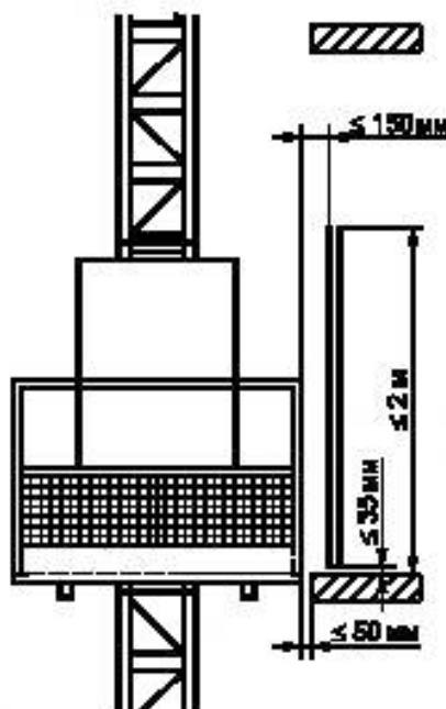
Рисунок 5 — Пример дверей погрузочной площадки в полную высоту
