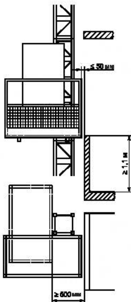
Рисунок 7 — Пример погрузочной площадки с неподвижным защитным устройством
