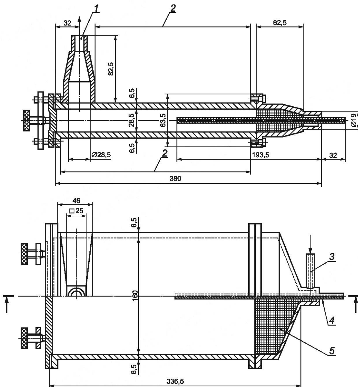
1 — выпускное отверстие для азота; 2 — пространство для нагревательного элемента; 3 — входное отверстие для азота; 4 — трубка для термометра; 5 — медная сетка с размером отверстий 0,25 мм
