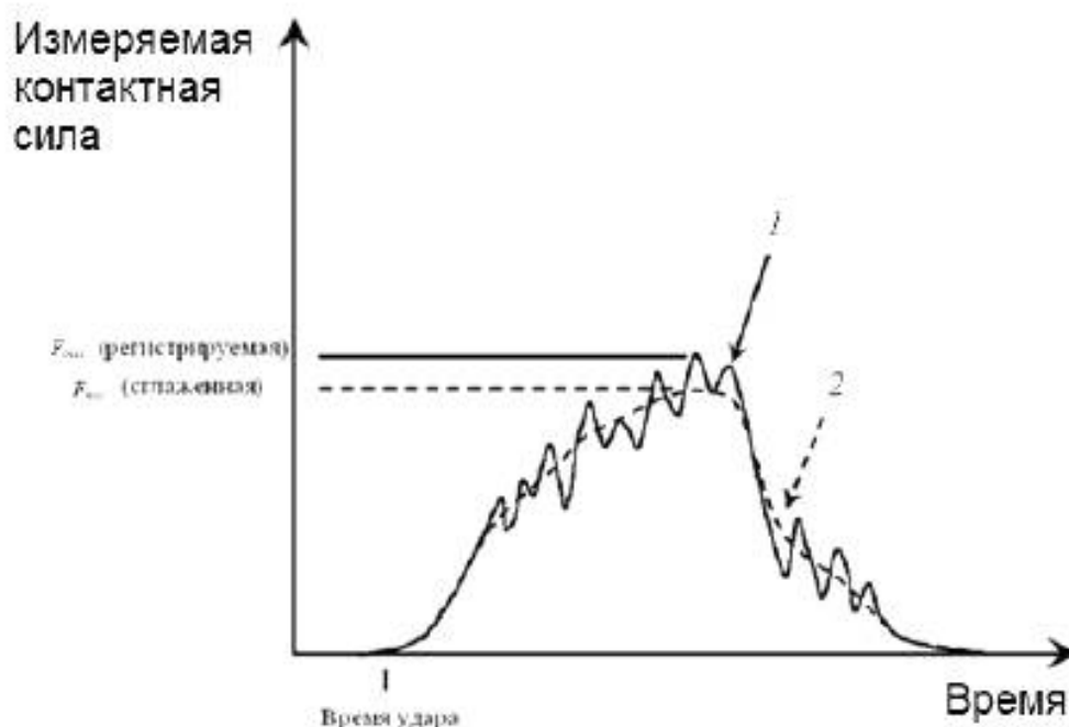
1 — регистрируемая кривая зависимости силы от времени при ударе с гармоническими колебаниями ударника, датчика силы и/или образца; 2 — сглаженная кривая зависимости силы от времени
