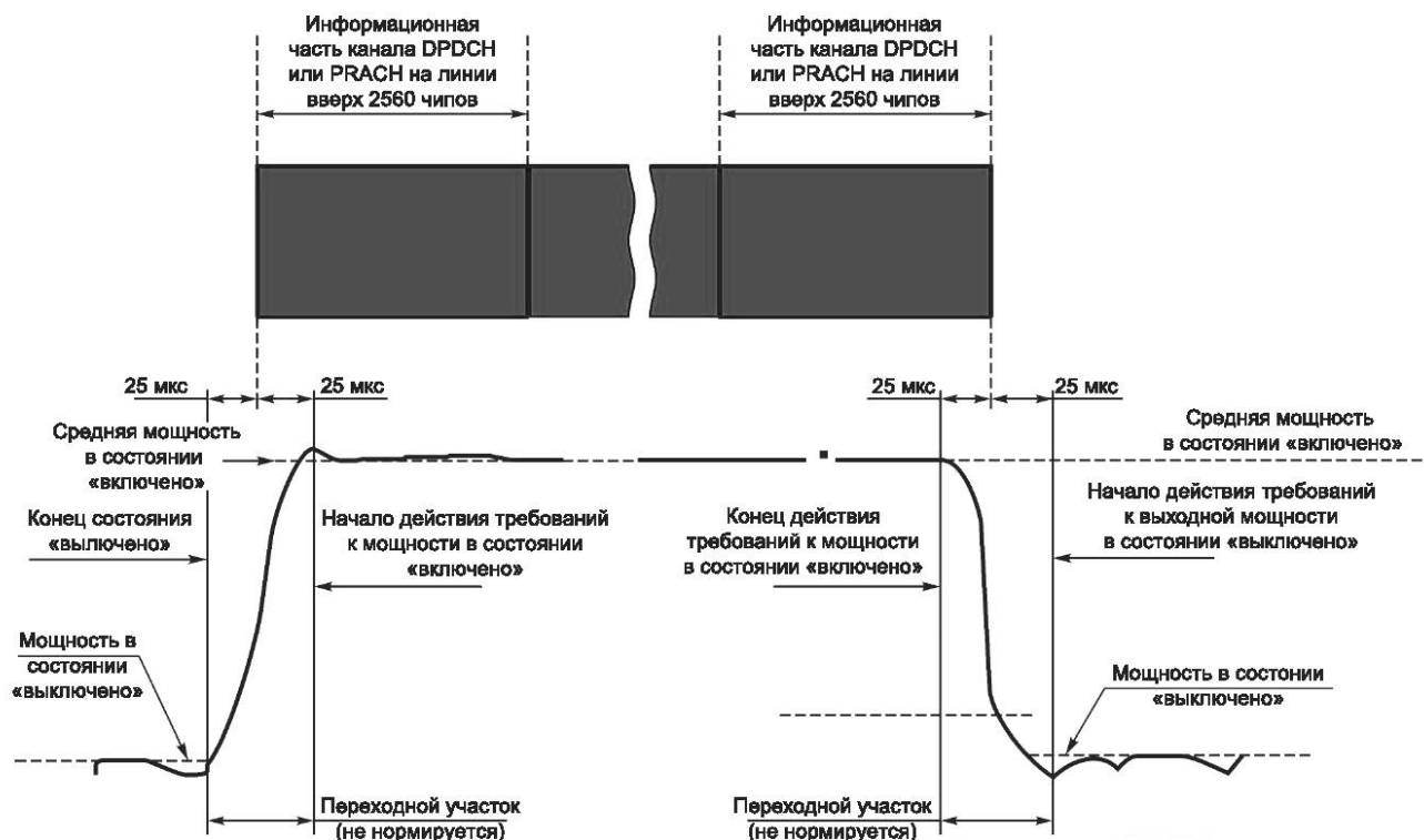
Рисунок В.2 — Шаблон включения и выключения излучения передатчика во времени для всех остальных каналов
