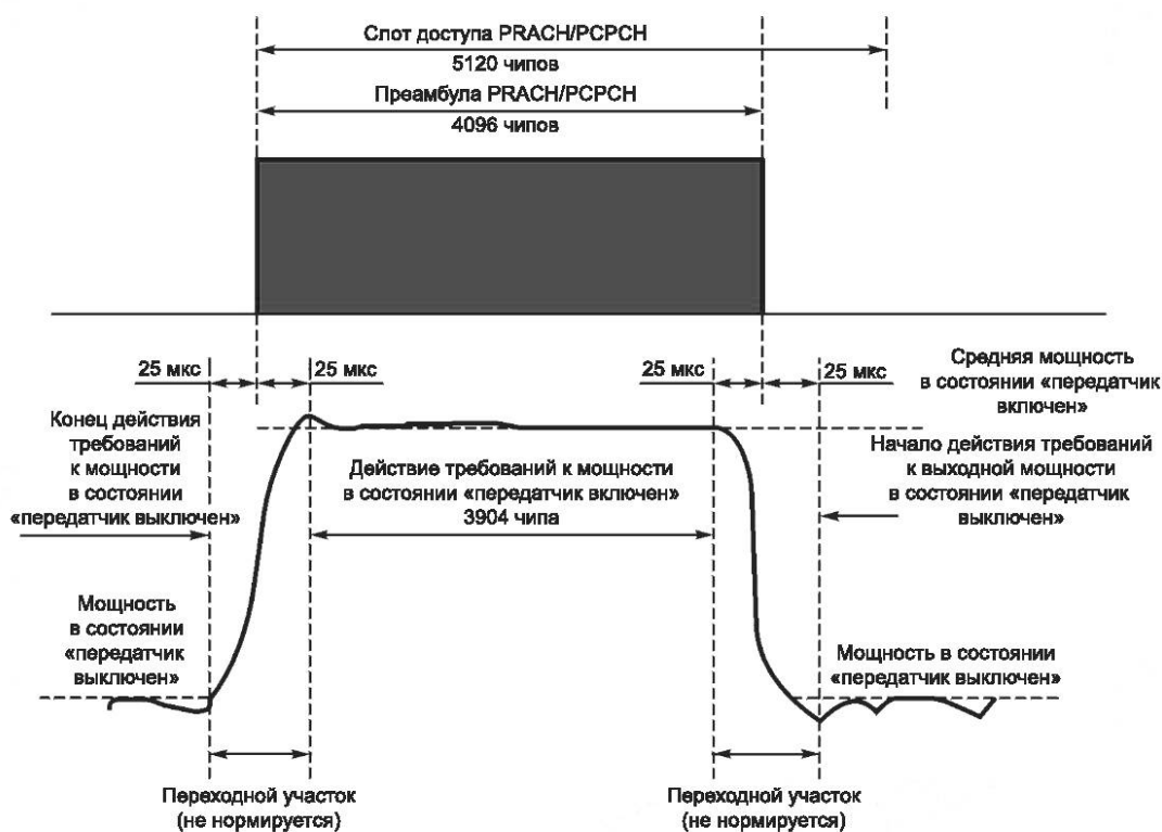
Рисунок В.1 — Шаблон включения и выключения излучения передатчика во времени для физического канала произвольного доступа
