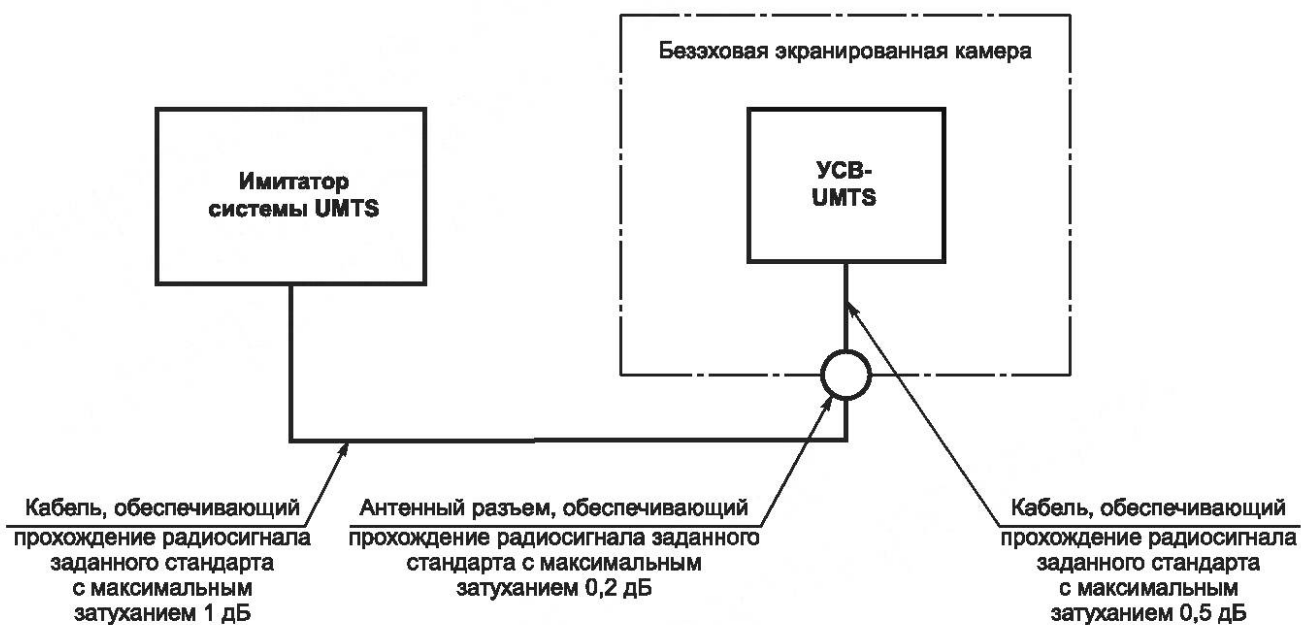
Рисунок Д.1 — Схема испытаний UCB-UMTS с использованием имитатора системы UMTS
