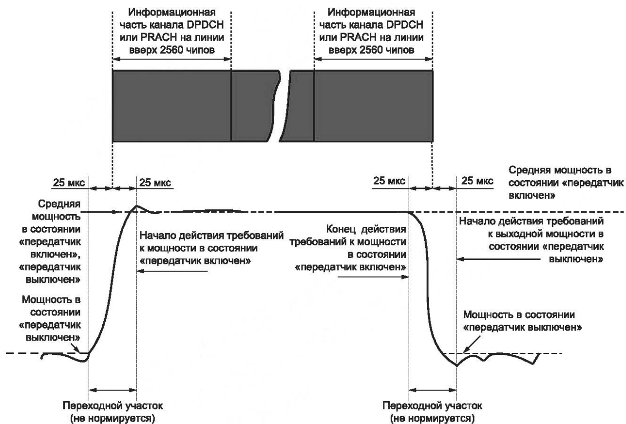
Рисунок 4 — Шаблон включения и выключения излучения передатчика во времени для всех остальных каналов
