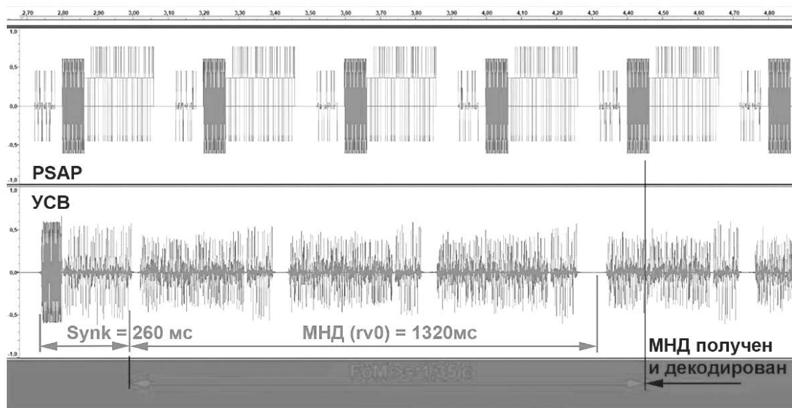
Рисунок 5 — Определение времени передачи МНД (FoM)
