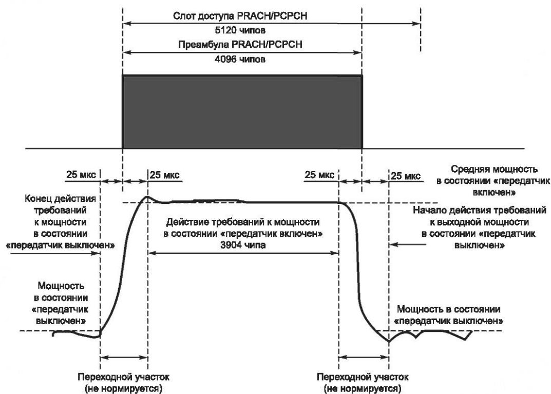
Рисунок Б.1 — Шаблон включения и выключения излучения передатчика модема UMTS 900 во времени для физического канала произвольного доступа
