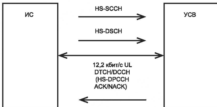
Рисунок Д.2 — Схема испытаний UCB-UMTS для определения предельно допустимой максимальной мощности в режиме HSDPA
