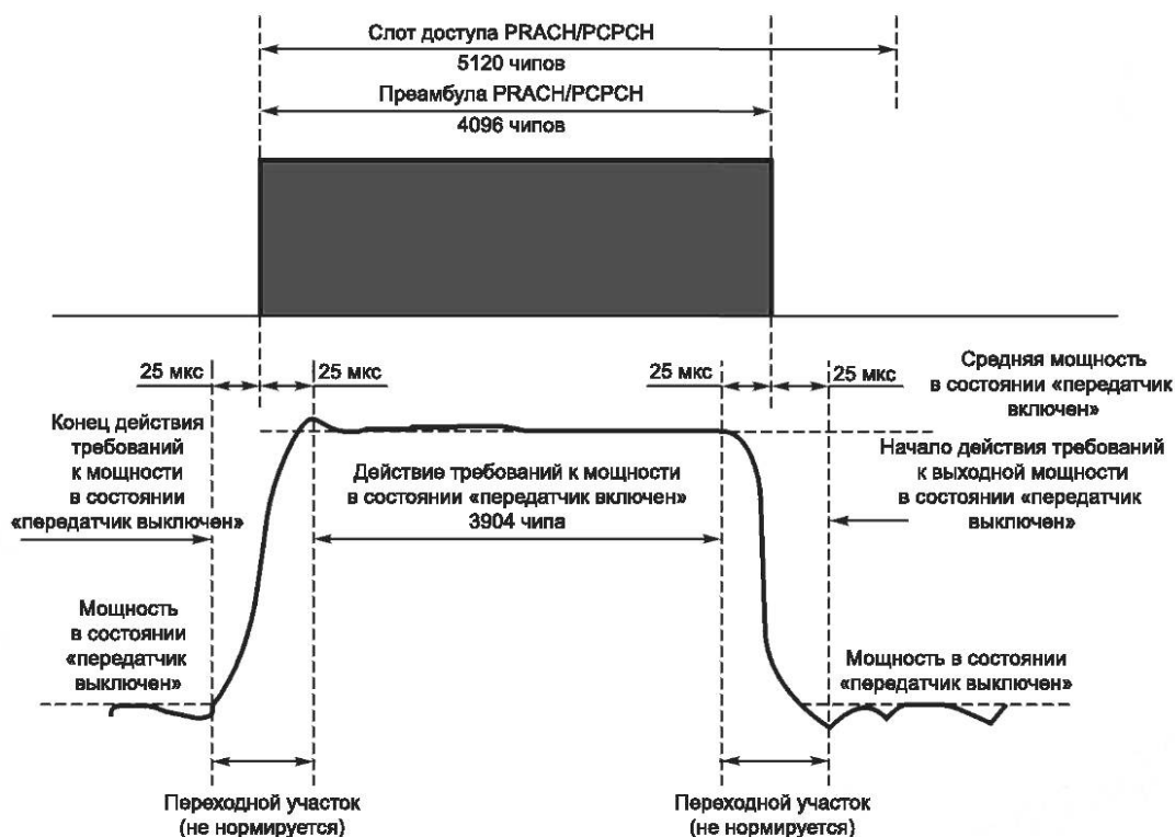
Рисунок 3 — Шаблон включения и выключения излучения передатчика во времени для физического канала произвольного доступа
