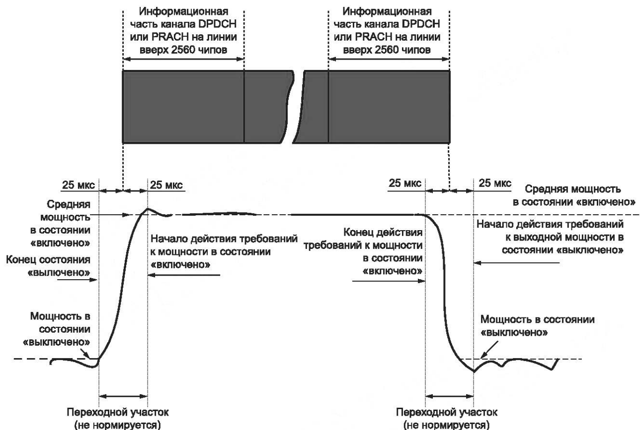
Рисунок Б.2— Шаблон включения и выключения излучения передатчика модема UMTS 900 во времени для всех остальных каналов
