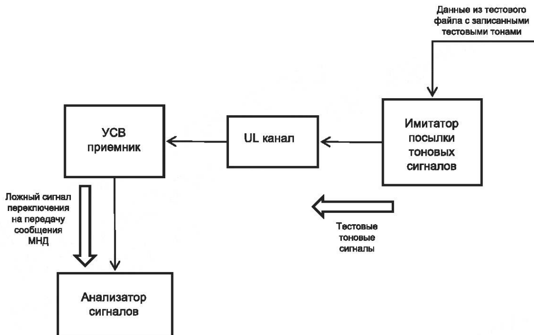
Рисунок Е.5 — Общая схема проведения проверки ложного детектирования экстренного вызова при наличии сигнальных тонов на входе приемника тонального модема
