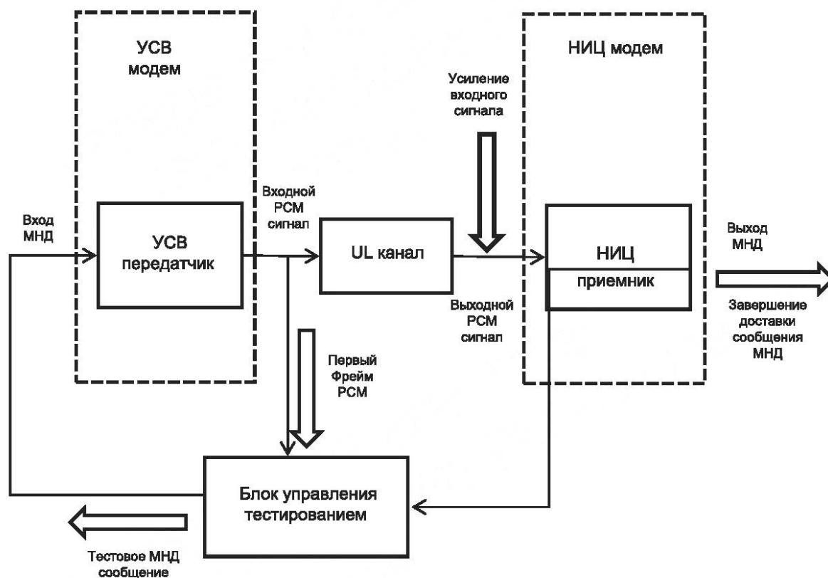
Рисунок Е.4 — Общая схема проведения тестирования при измерении времени передачи сообщения МНД при различных значениях коэффициента усиления PCM сигнала
