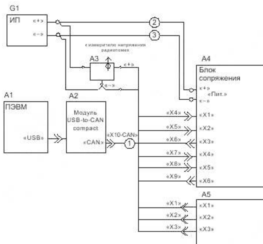
А1 — ПЭВМ; А2 — модуль USB-to-CAN; А3 — V-образный эквивалент сети (см. таблицу 2); А4 — блок сопряжения; А5 — испытываемая УСВ; G1 — источник питания; L1 — катушка индуктивности с воздушным сердечником, рассчитанная на ток до 5 А; P1 — осциллограф; 1 — кабель; 2, 3 — провод ML-4G
