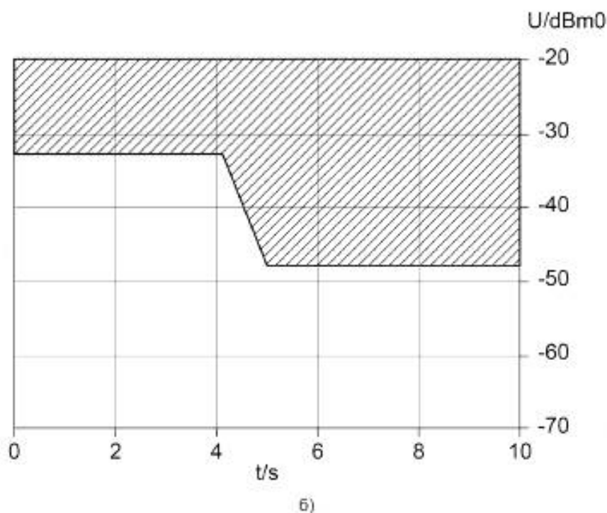
Рисунок И.1 — Зависимость степени подавления экосигналов L и уровня экосигналов U от времени
