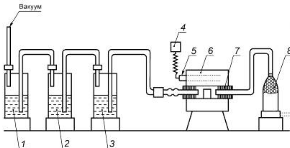
1—3 — склянки Дрекслея поглотительные; 4 — терморегулятор; 5 — термолара; 6 — печь трубчатая электрическая; 7 — лодочки фарфоровые; 8 — склянка Тищенко СПТ
