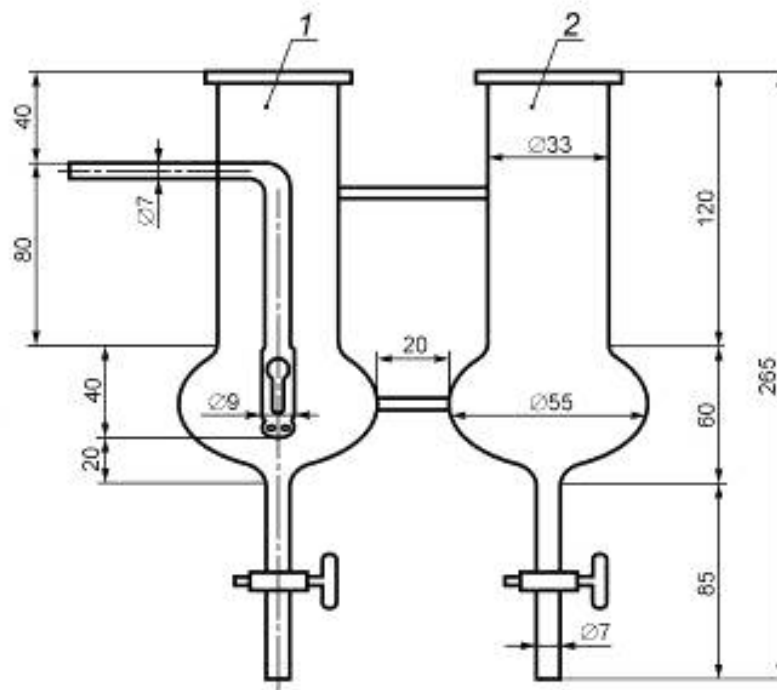
Рисунок 2 — Устройство поглотительного сосуда
