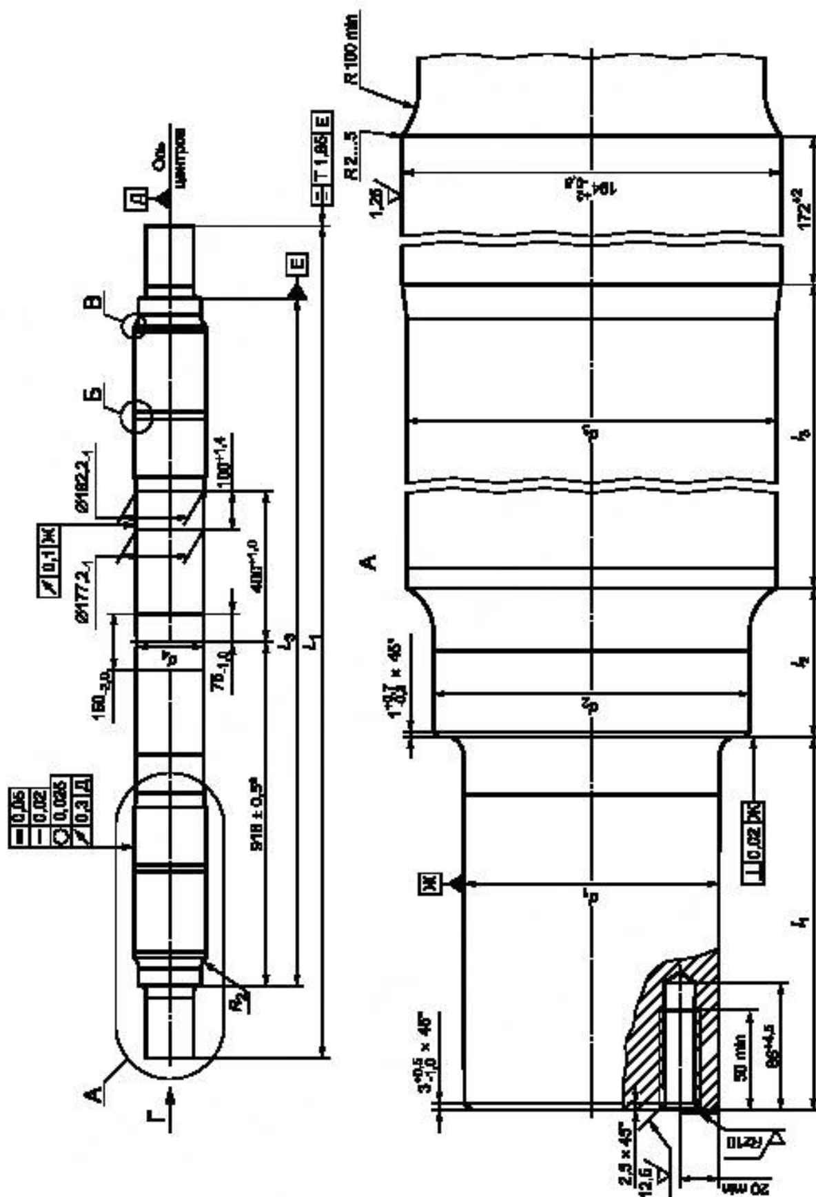
Рисунок А.5, лист 1 — Ось типа RB3Ш для пассажирских вагонов локомотивной тяги, СПС
