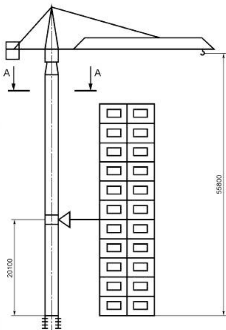
Рисунок 1 — Пример схемы расположения опорного крепления на кране
