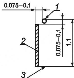
1 — поручень; 2 — боковое ограждение; 3 — пол (настил) кабины (люльки)
