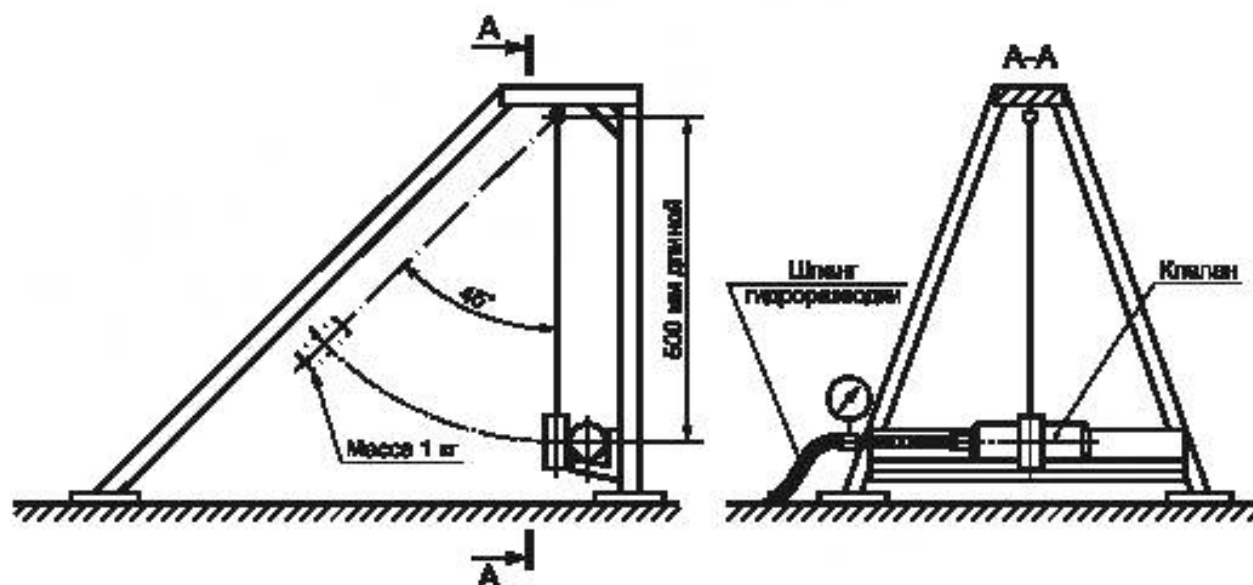
Рисунок А.3 — Испытание на ударную прочность
