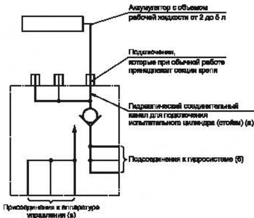
Рисунок А.5 — Испытательный контур для гидрозамков
