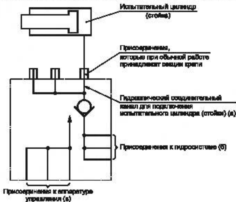
Рисунок А.4 — Испытательный контур для гидрозамков
