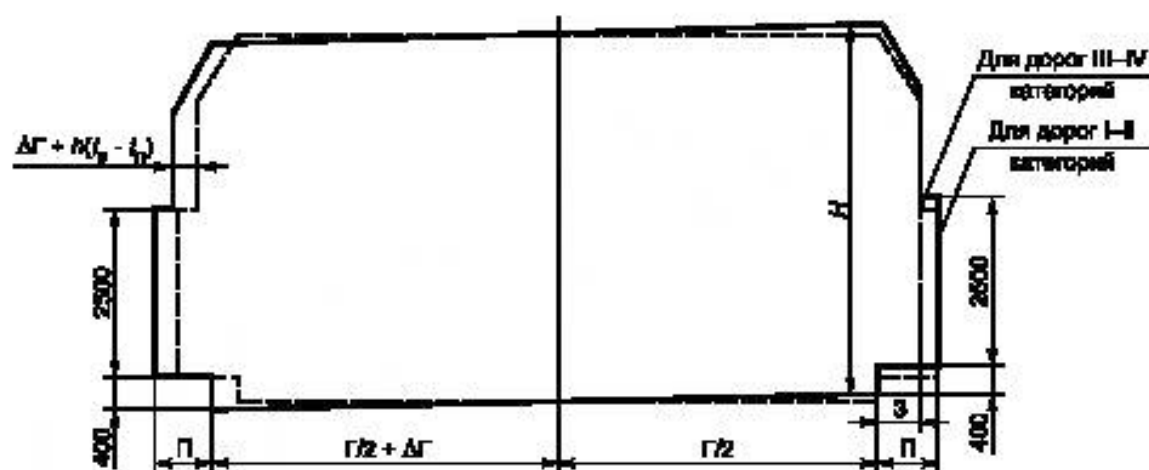
\Gamma — габарит по ширине; \Delta\Gamma — величина уширения габарита; H — габарит по высоте тоннеля; h — высота автотранспортного средства; i_n, i_p — поперечные уклоны проезжей части на вираже и на прямой
