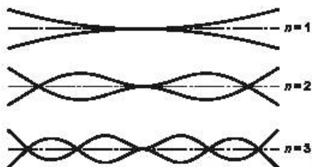
Рисунок 1 — Примеры мод колебаний
