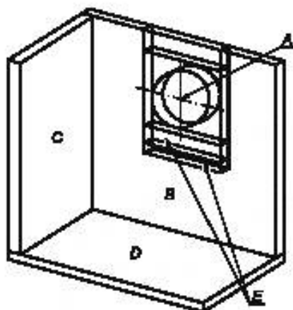
А — осевая линия дымохода; В — задняя стенка; С — боковая стенка; D — пол испытательного угла; Е — вставки
