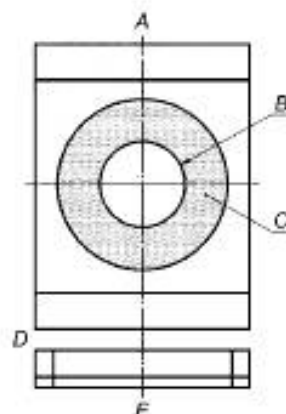
А — вид спереди; В — дымоход; С — теплоизоляция, расстояние (150 \pm 5) мм до дымохода, заполненное изоляционным материалом; D — аналогично конструкции на рисунке А.3; Е — вид сверху
