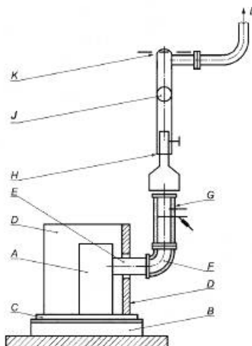
Рисунок А.1 — Пример типовой установки отопительного прибора с вертикальным отводом дымовых газов в схеме испытаний
