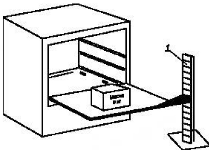
1 — датчик с измерительной линейкой
