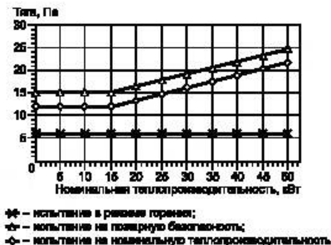
Рисунок 1 — Значения тяги в дымоходе
