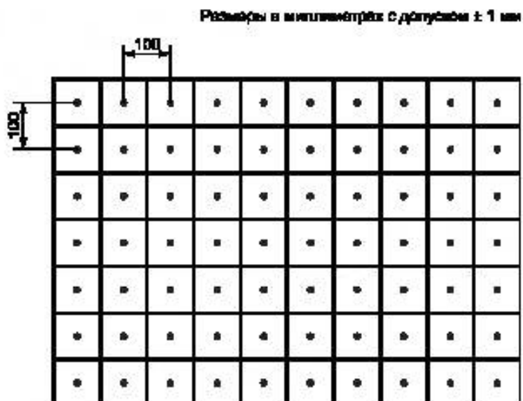
Рисунок А.6 — Вид сверху пола и стенок испытательного угла с расположением измерительных точек размеров в миллиметрах
