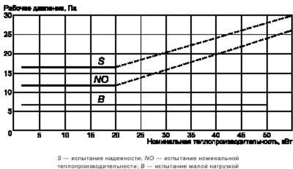
Рисунок 1 — Значения рабочего давления
