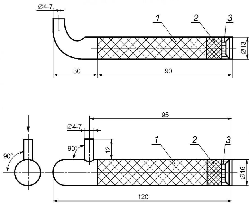
Рисунок Г.1 — Фитровальные патроны
