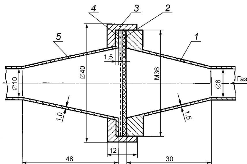
Рисунок Д.4 — Держатель для фильтров АФА
