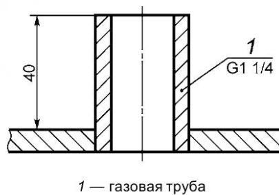
Рисунок Б.3 — Штуцер для измерения давления газа
