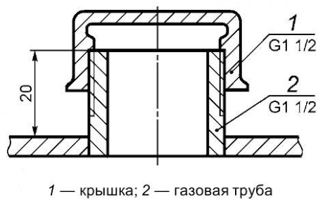
Рисунок Б.1 — Штуцер для измерения скорости и запыленности газа
