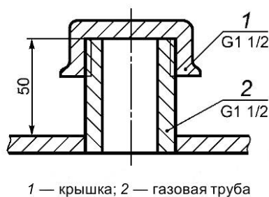
Рисунок Б.2 — Штуцер для измерения температуры газа
