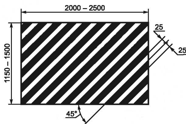
Рисунок 1 — Экран «зебра»
