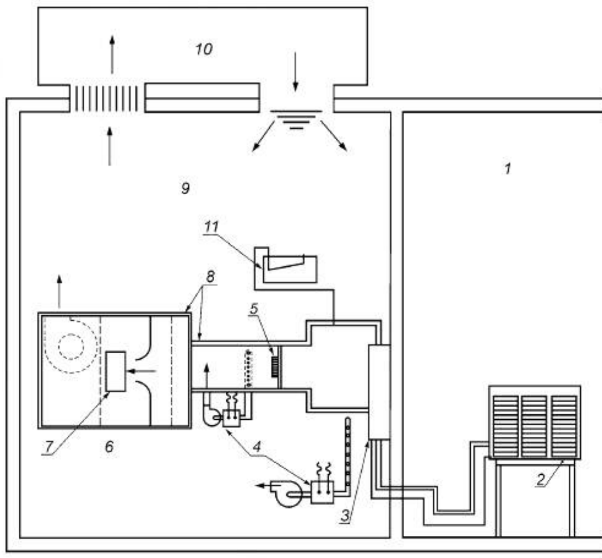
1 — отсек наружной стороны; 2 — наружный блок испытываемого оборудования; 3 — секция испытываемого оборудования с внутренним теплообменником; 4 — измерительные приборы температуры и влажности; 5 — смеситель; 6 — аппаратура измерения воздушного потока; 7 — дверь/окно; 8 — изоляция; 9 — отсек внутренней стороны; 10 — аппарат кондиционирования помещения; 11 — аппаратура для измерения перепада давления
