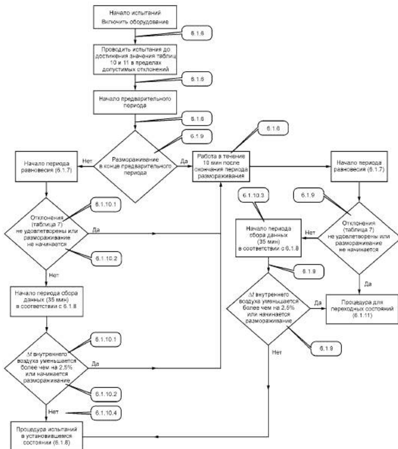
Рисунок Н.1 — Блок-схема процедуры
