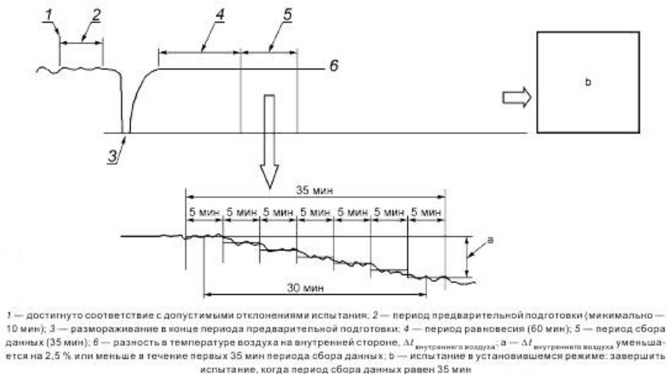
Рисунок Н.2 — Испытание теплопроизводительности в установившемся режиме
