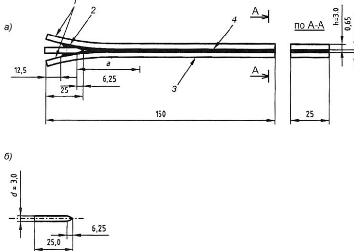
1 – начальное расслоение контрольного образца-пластины на 12,5 мм; 2 – клин для испытаний; 3 – заготовка (часть изделия) – пластина размером 150х25х3 мм; 4 – клеевой шов толщиной 0,65 мм
