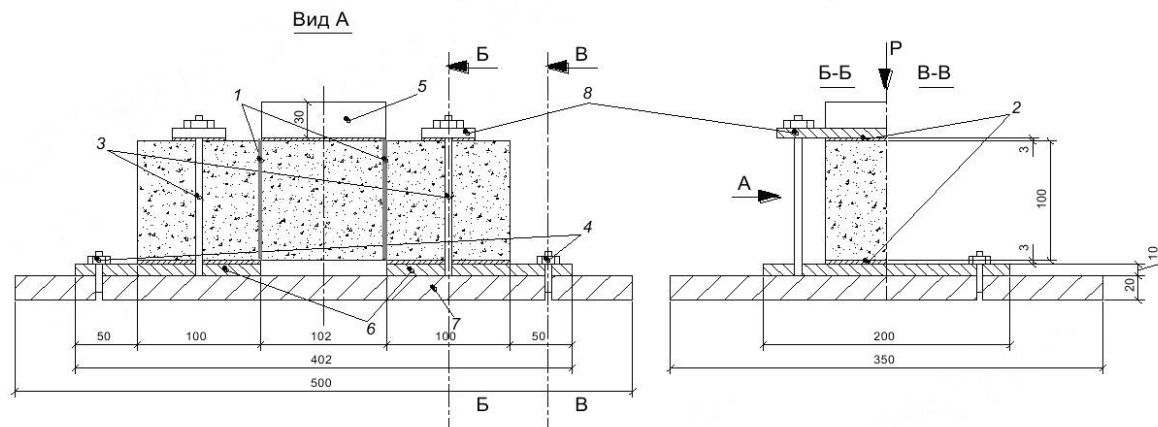
Рисунок В.2 – Кондуктор для крепления при испытании контрольных образцов-призм размером 100х100х302 мм с вертикальными клеевыми швами
