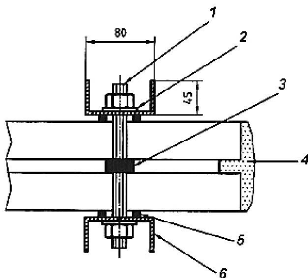
Рисунок Д.2 – Сборный образец-плита в кондукторе для формирования зазора (клеевого шва) – вид спереди
