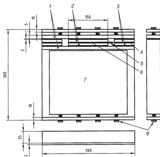
1 – стальная полоса-подкладка; 2 – заготовки (части изделия) – пластины размером 150х25х3 мм; 3 – прокладка толщиной 3 мм; 4 – прокладка толщиной 0,65 мм; 5 – шаблон-вставка с лентой ПВХ для создания непроклеенного зазора в виде петли на глубину 12,5 мм; 6 – создаваемый клеевой шов; 7 – стальной блок-основание; 8 – винты крепления
