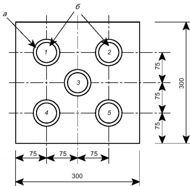
Рисунок В.3 – Схема разметки и маркировки мест бурения образцов-кернов диаметром (50 \pm 0,5) мм в сборно-монолитном образце-плите
