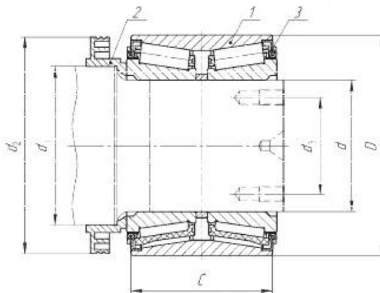
1 – базовый подшипник; 2 – лабиринтное кольцо; 3 – уплотнение
