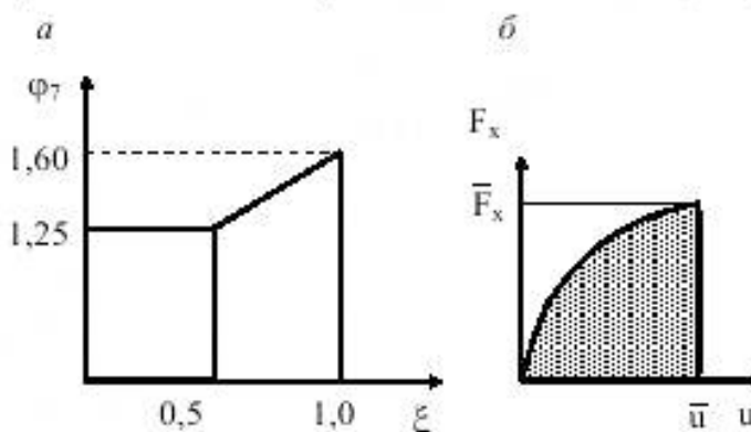
Рисунок 5 – Схемы к расчету коэффициента \varphi_7
