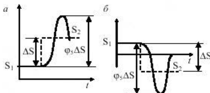
Рисунок 3 – Схемы к расчету коэффициента \varphi_5 . Пунктиром показан график изменения движущей силы привода.
