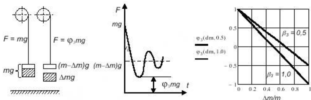
Рисунок 2 – Схемы к определению коэффициента \varphi_3
