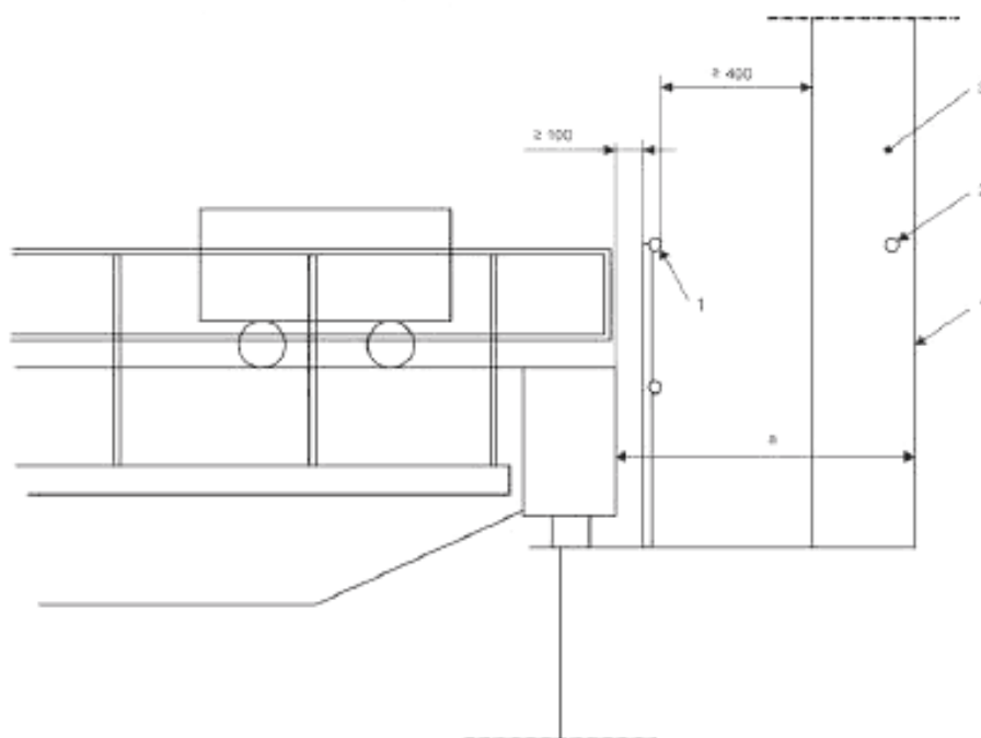
1 – перила А; 2 – перила Б; 3 – колонна; 4 – стена
