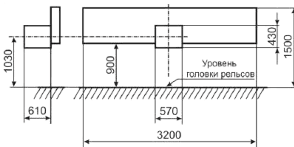
Рисунок 2 – Размеры препятствия при аварийном столкновении по сценарию 2
