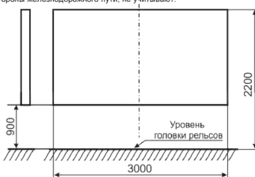
Рисунок 1 – Размеры препятствия при аварийном столкновении по сценарию 1
