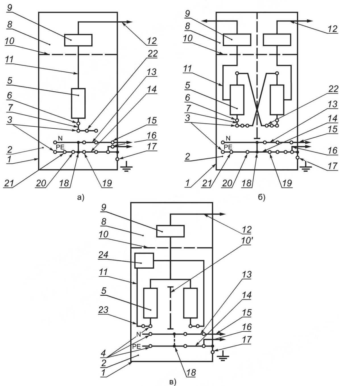
Рисунок Б.1, лист 1 — Схемы расположения аппаратуры в вводных панелях многопанельных ВРУ: а) с одним вводом; б) с двумя вводами; в) с двумя взаиморезервируемыми вводами с аппаратурой АВР
