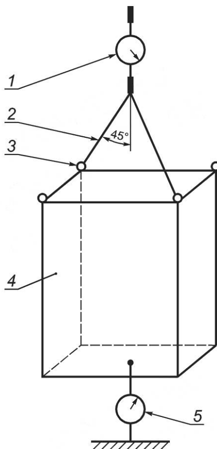
1 — динамометр 1; 2 — трос; 3 — строповое устройство; 4 — ВРУ; 5 — динамометр 2
