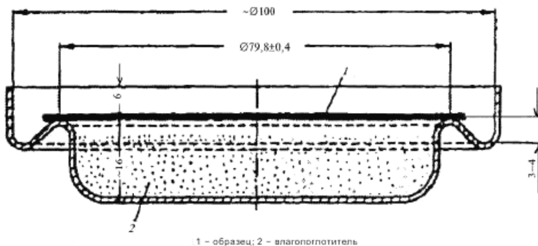
Рисунок 1 – Алюминиевая чашка с влагопоглотителем
