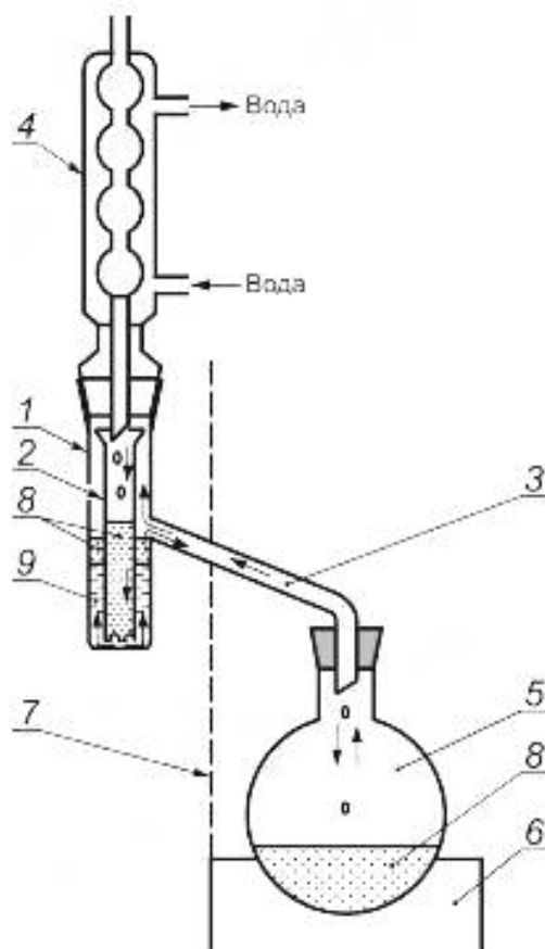
1 — пробирка со шпифом; 2 — трубка с расширением, вставляемая в пробирку 1; 3 — боковой отвод; 4 — холодильник; 5 — экстракционная колба; 6 — колбонагреватель (электроплитка); 7 — теплоизолирующий экран; 8 — диэтиловый эфир; 9 — водная вытяжка пробы
