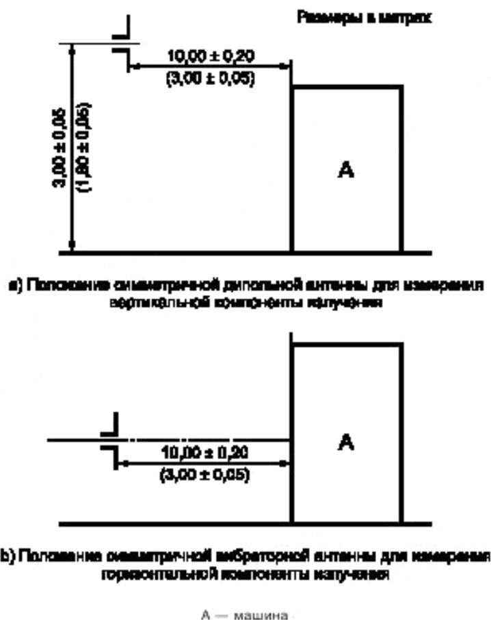
Рисунок В.2 — Расположение антенны относительно машины при измерениях
