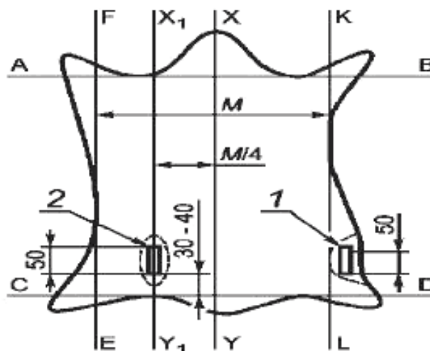
Рисунок 4 - Схема расположения образцов для определения температуры сваривания
