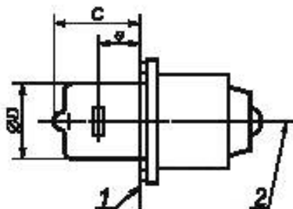
1 – базовая плоскость; 2 – базовая ось
