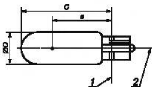
1 – базовая плоскость, 2 – базовая ось
