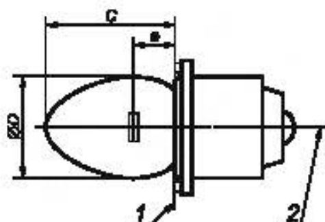
1 – базовая плоскость. 2 – базовая ось
