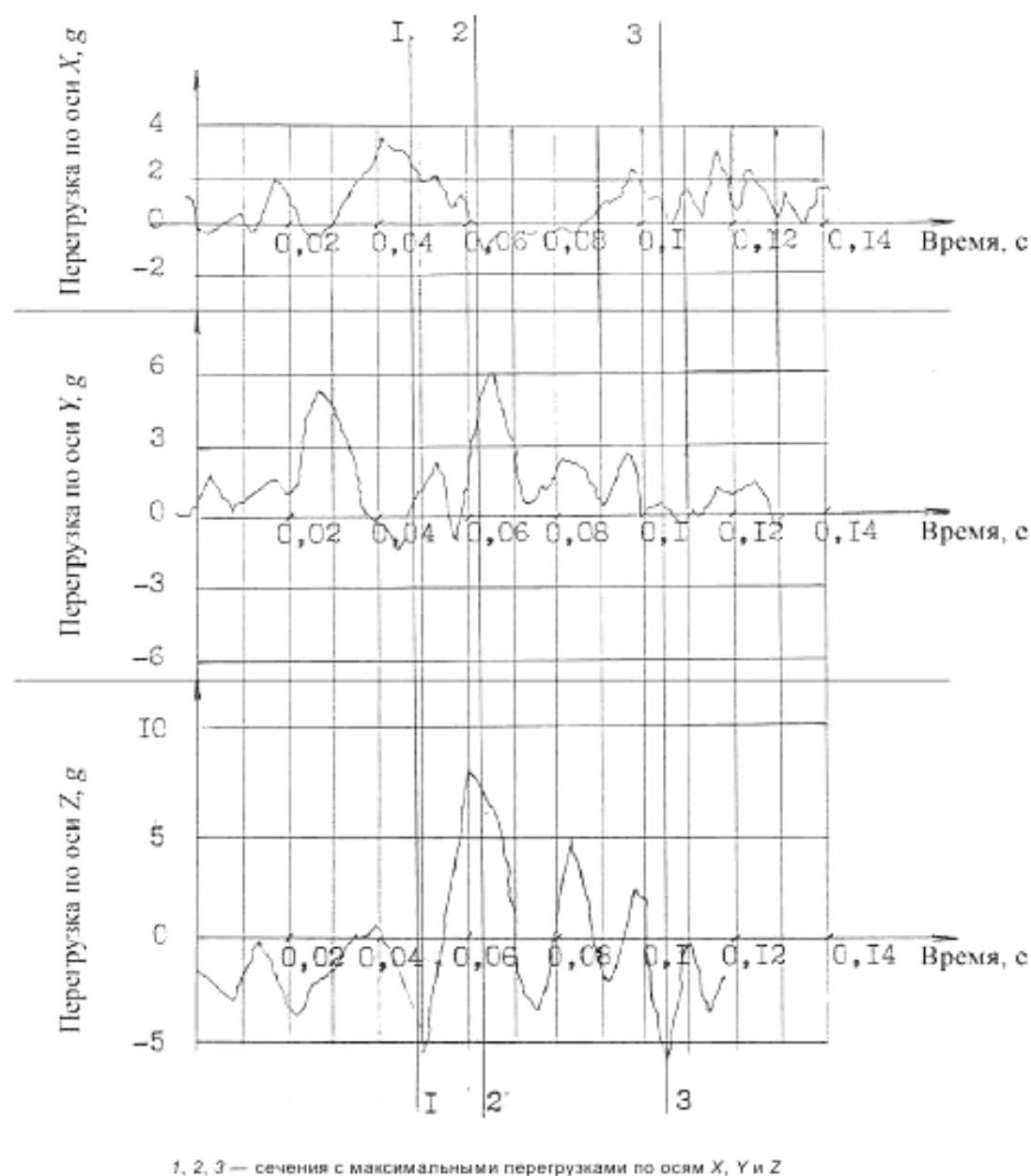
Рисунок 7 — Пример совмещенной диаграммы ускорений (перегрузок) в центре масс автомобиля по осям X, Y и Z
