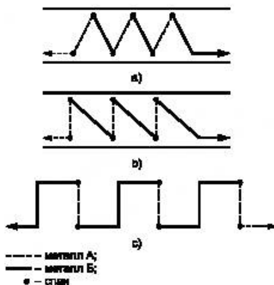
Рисунок D.7 — Примеры расположения спаев термодатчиков термобатареи
