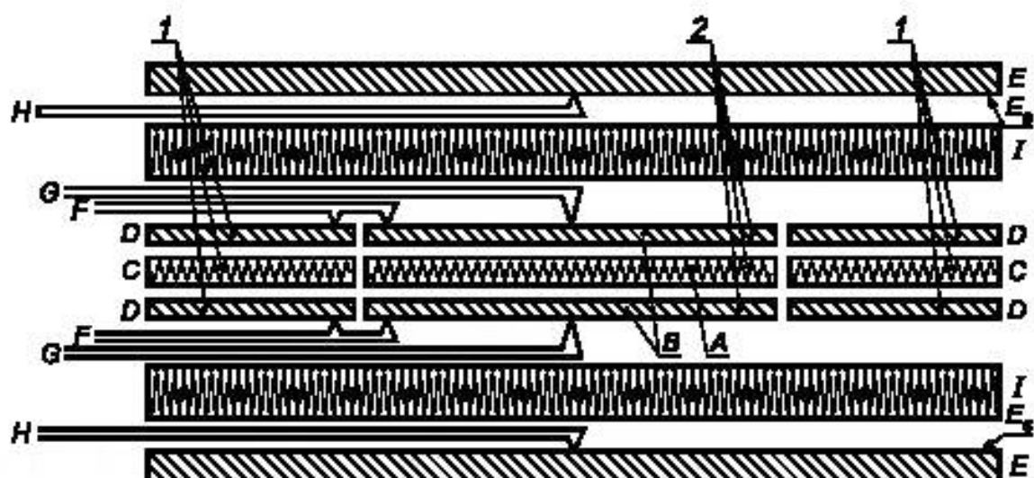
а) Прибор для одностороннего испытания двух образцов
