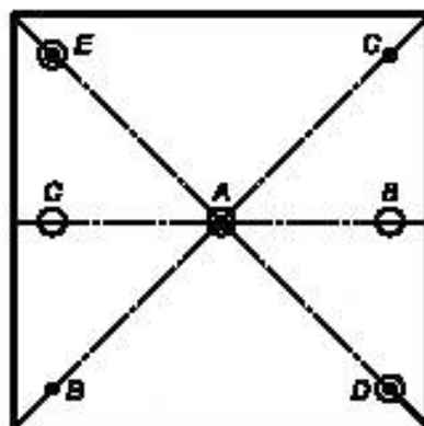
Рисунок D.4 — Расположение термодпар на рабочих поверхностях плит нагревателя и холодильника
