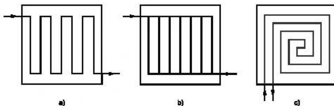
Рисунок D.6 — Схемы конструктивных решений трубок холодильника
