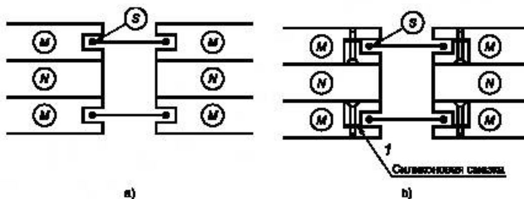
Рисунок D.3 — Конструктивное решение зазора
