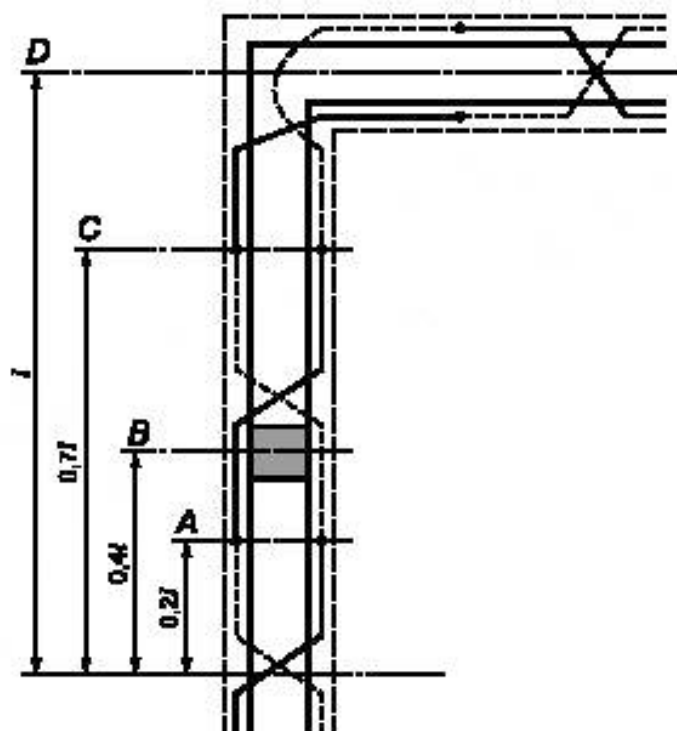
Рисунок D.2 — Расположение слейсера (прокладки) и спаев проводов уравнивающей термобатареи
