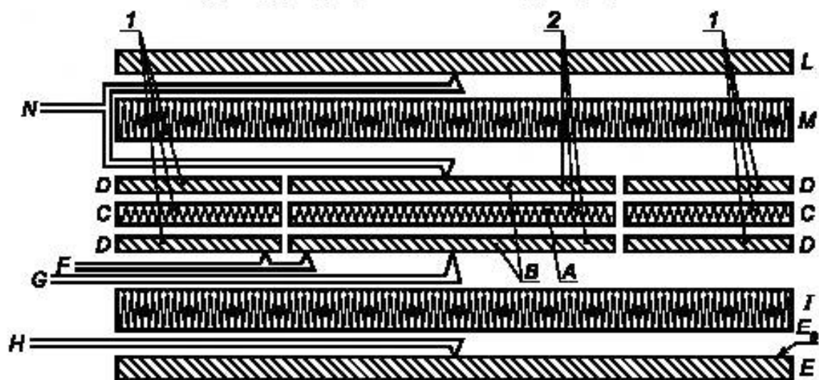
б) Прибор для испытания одного образца
