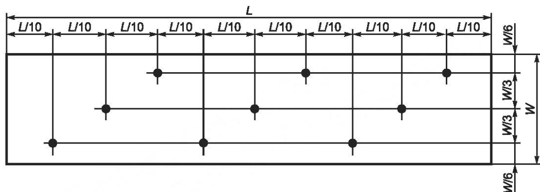
Рисунок 12 — Положение точек отбора проб на открытой поверхности железнодорожной платформы
