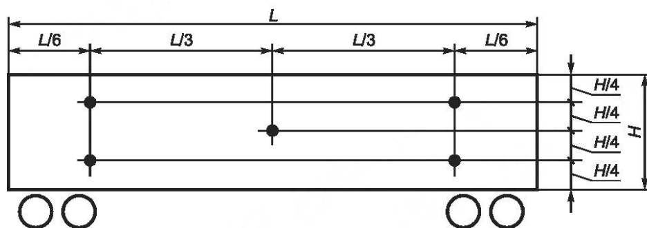
L — длина платформы; H — высота платформы
