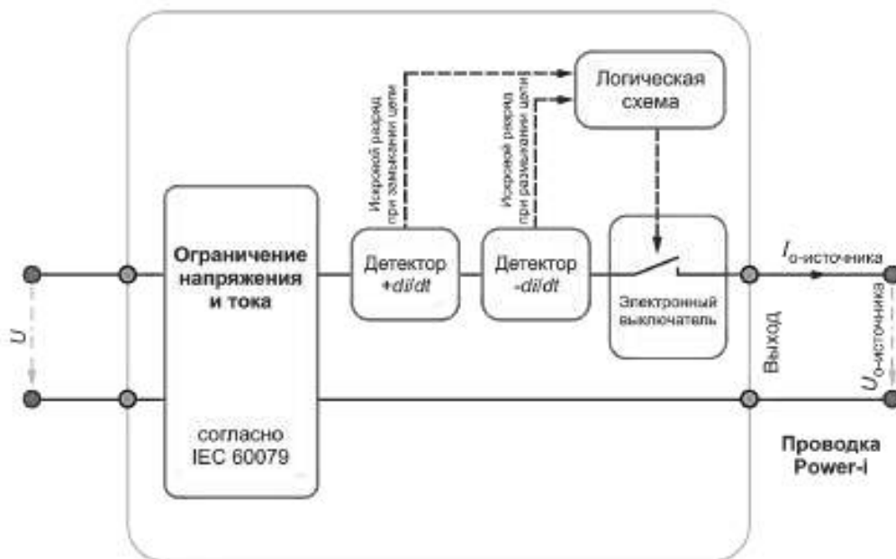
Рисунок 3 — Элементы источника Power-i с ограничением напряжения и тока
