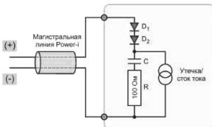
Рисунок С.5 — Пример ограничителя Power-i
