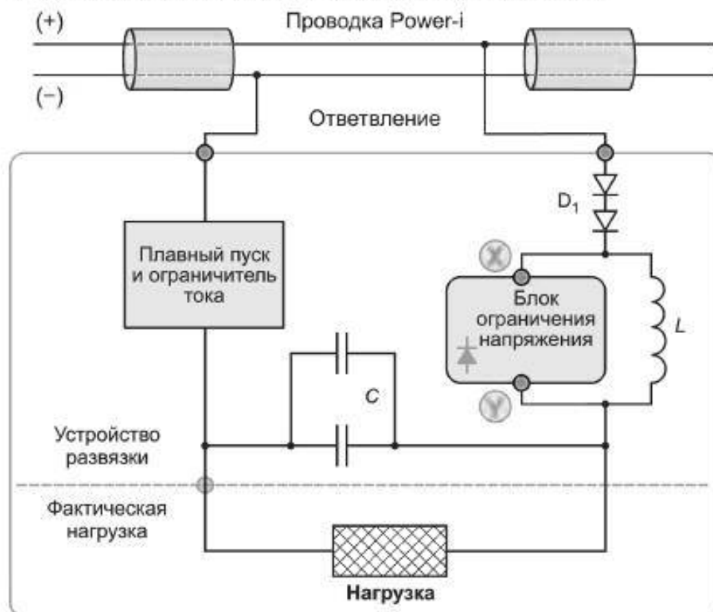
Рисунок С.2 — Пример обычного полевого устройства Power-i
