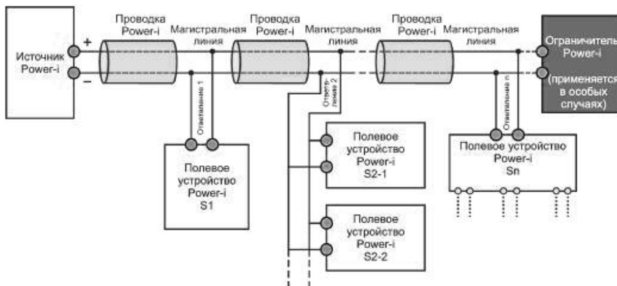
Рисунок 2 — Пример системы Power-i со сложной структурной схемой
