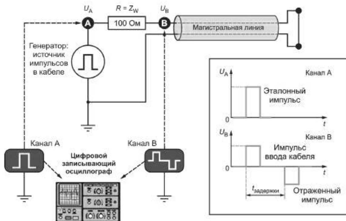
Рисунок А.13 — Испытательное оборудование для определения времени отклика магистральной линии Power-i (базовый принцип) t_{\text{отклика магистр. линии}}
