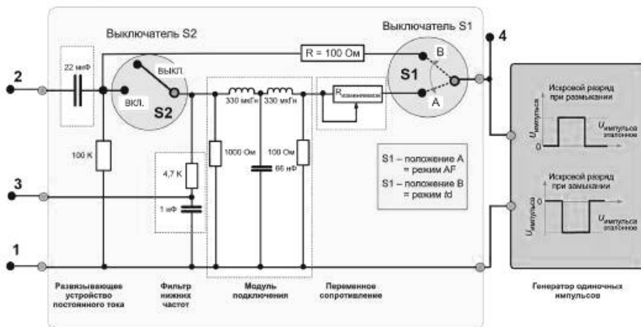
Рисунок А.1 — Базовые принципы универсального контрольно-испытательного оборудования Power-i
