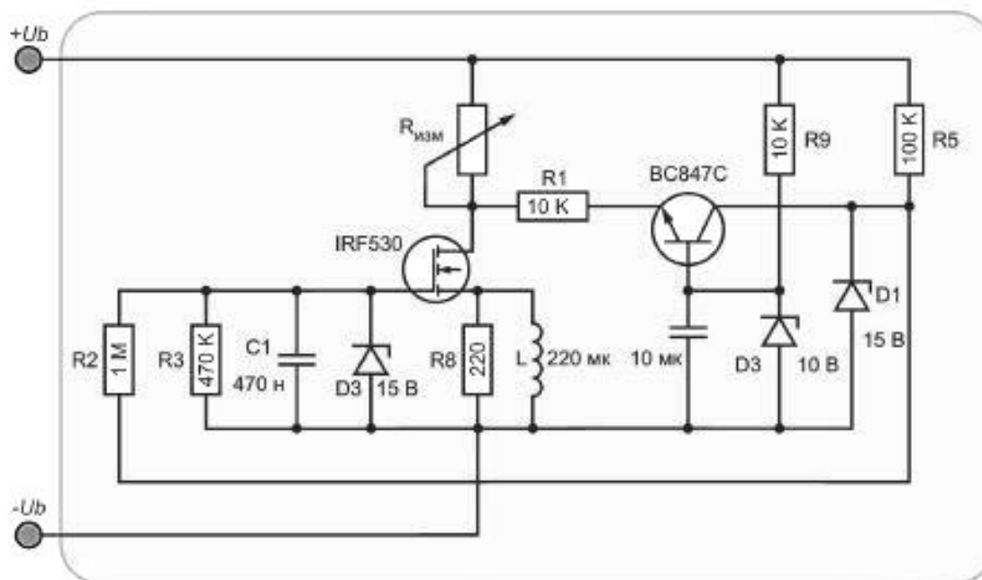
Рисунок С.4 — Искусственная нагрузка Power-i
