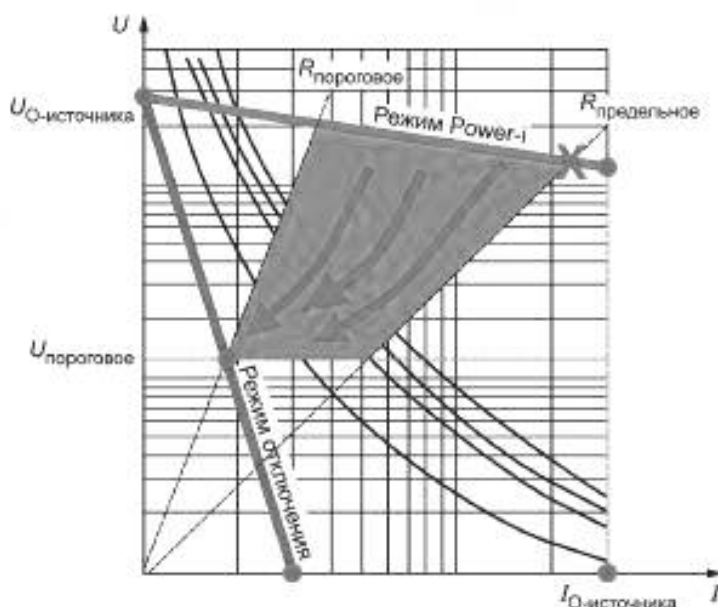
Рисунок В.5 — Набор выходных значений характеристических кривых источника Power-i при повреждении
