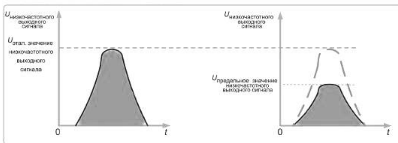
Рисунок А.2 — Импульс на выходе. Выводы 3 и 1 (см. рисунок А.1)
